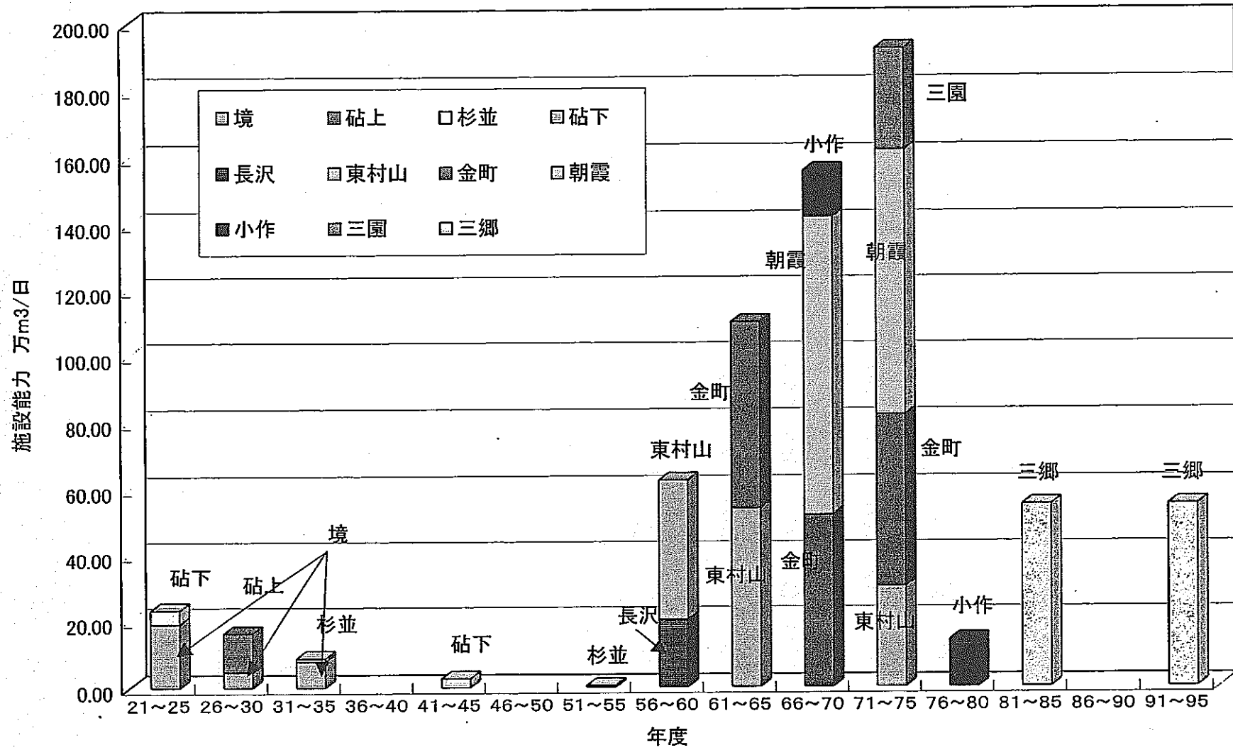
浄水場の建設年次別施設能力 (東京都水道局)
