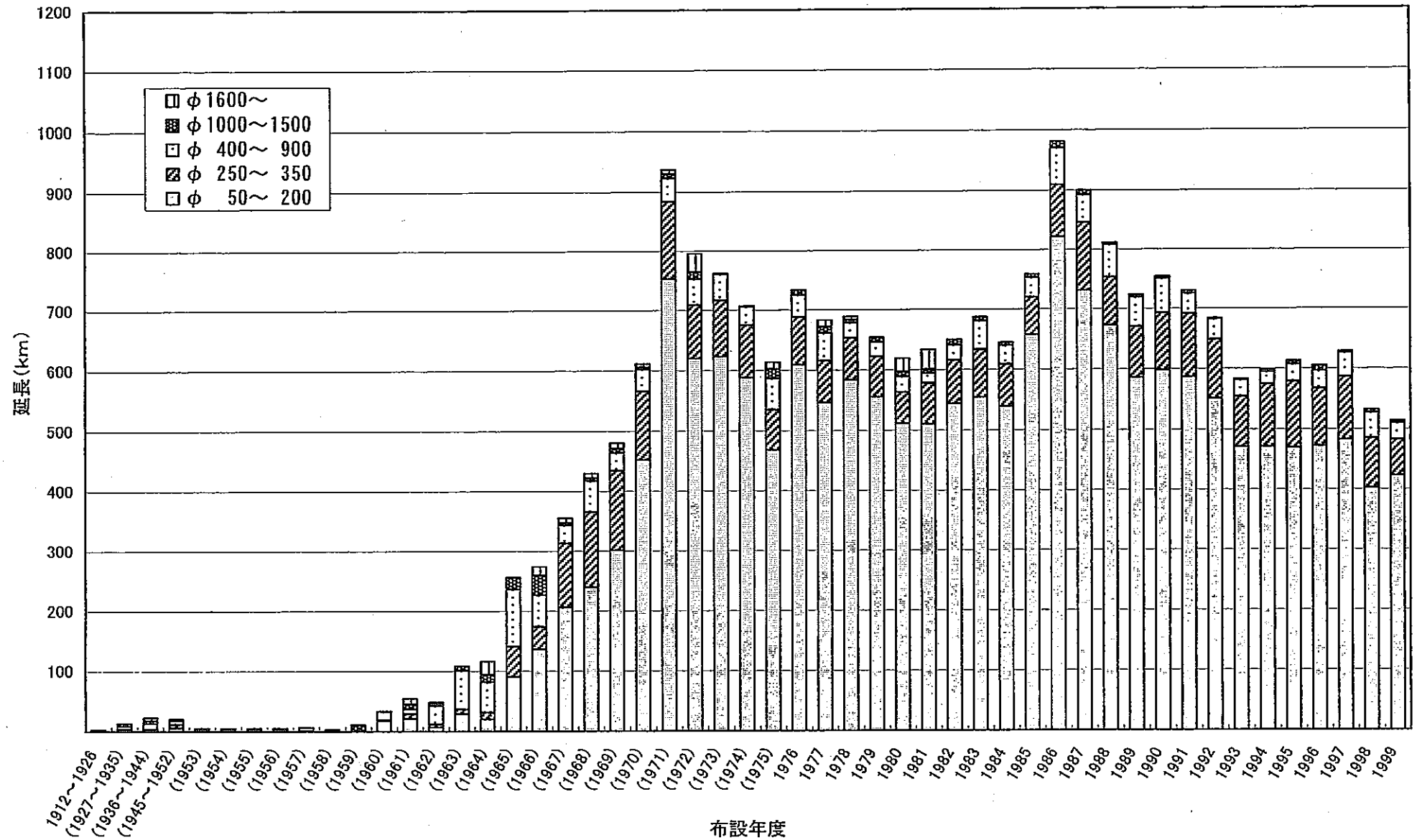
送水・配水管(本管+小管)布設年度別状況図〔区部+多摩〕(東京都水道局)
