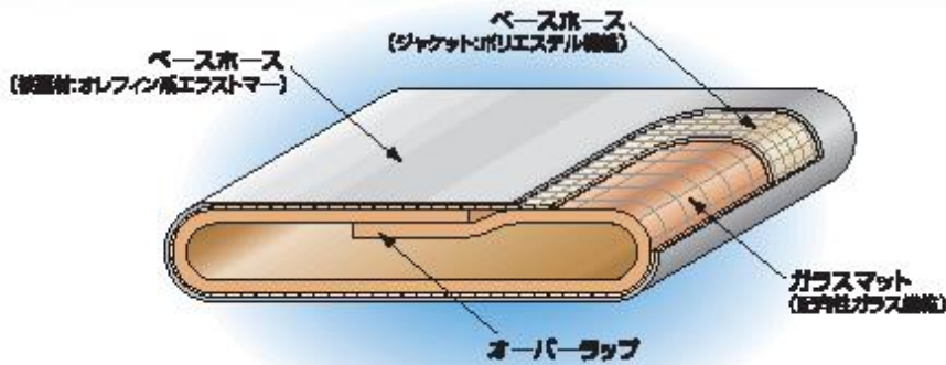
更新工法材料構造図
