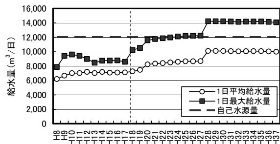
図Ⅳ-2.3 水需要予測(受水団体別)
