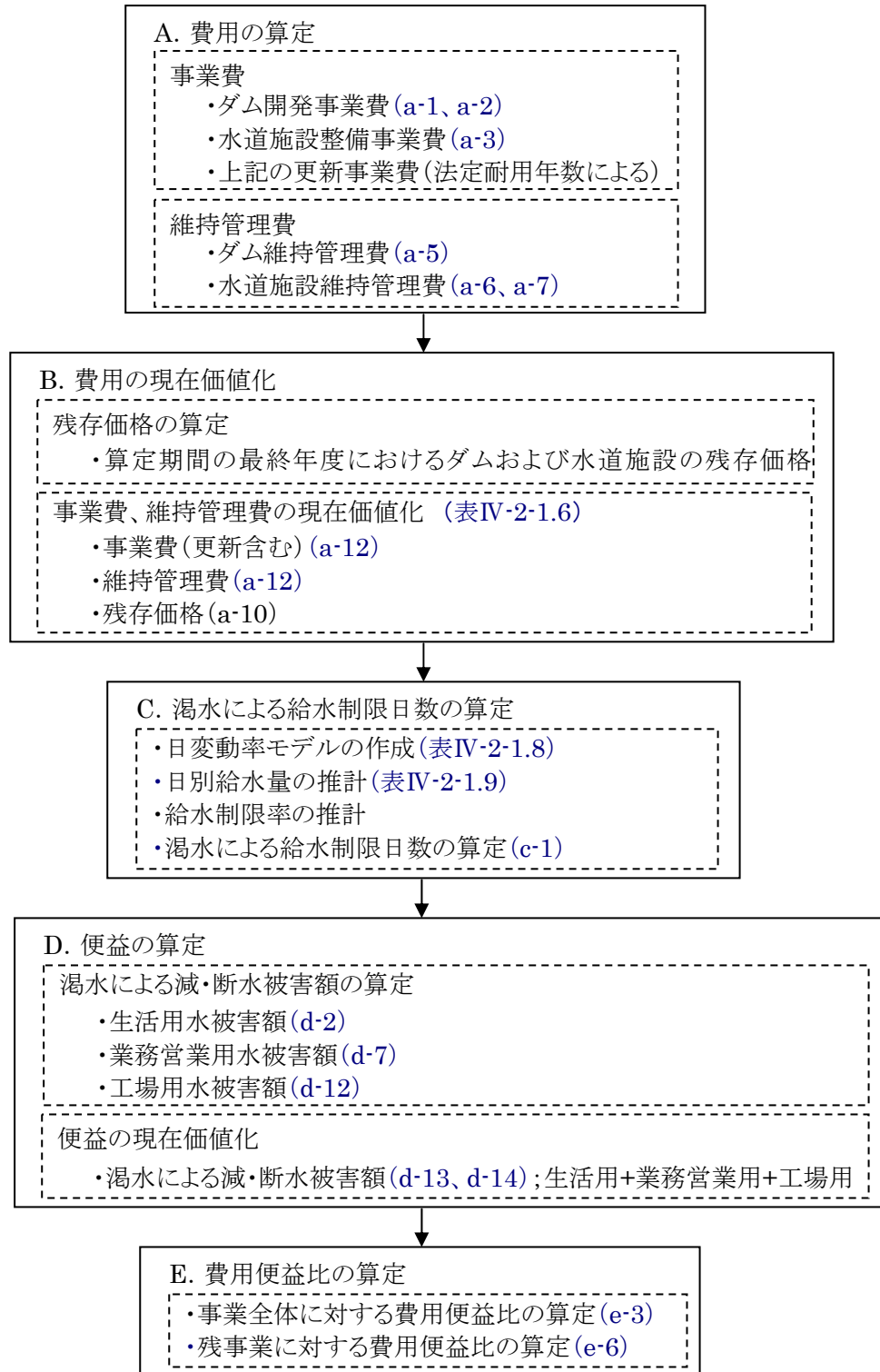
図Ⅳ-2-1.2 費用便益比の算定フロー
