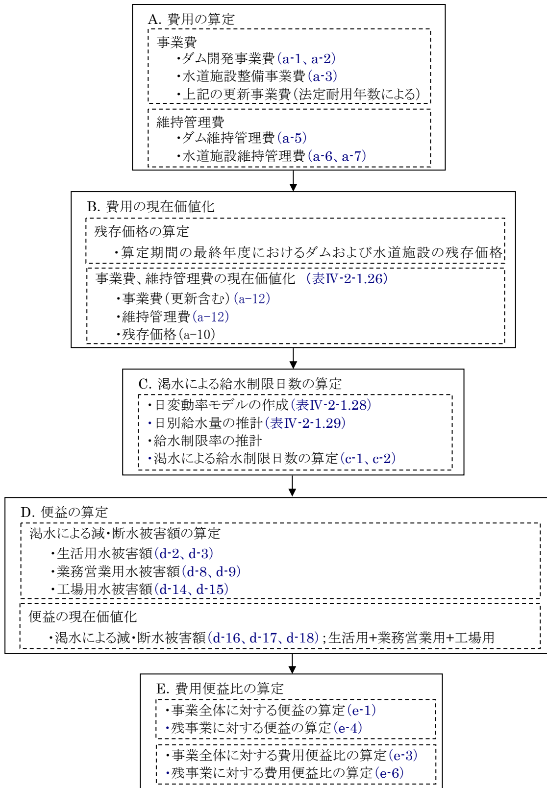
図Ⅳ-2-1.6 費用便益比の算定フロー
