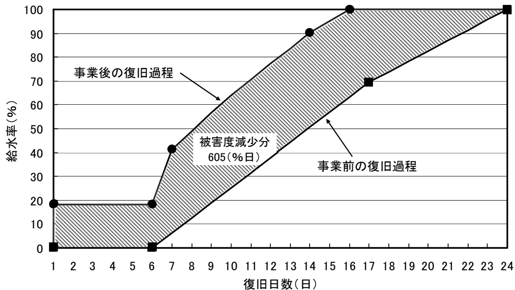
図Ⅳ-2-1.9 地震発生時の復旧過程
