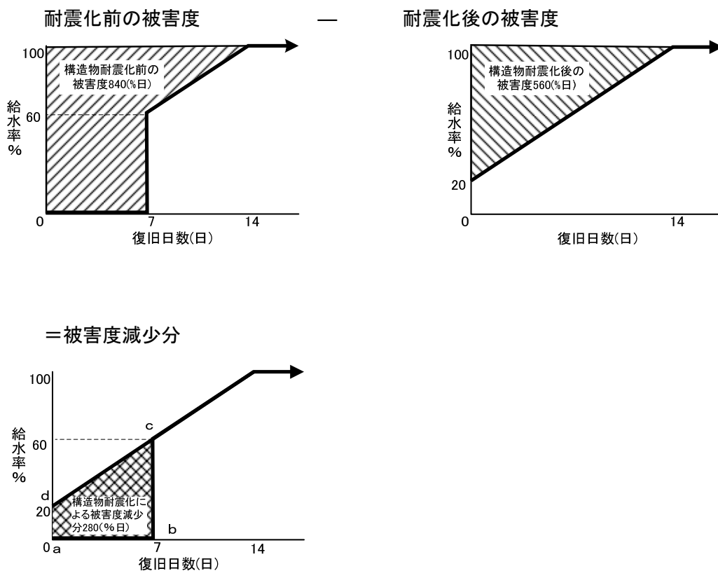
図Ⅳ-1-3.10 被害度減少分の算定
