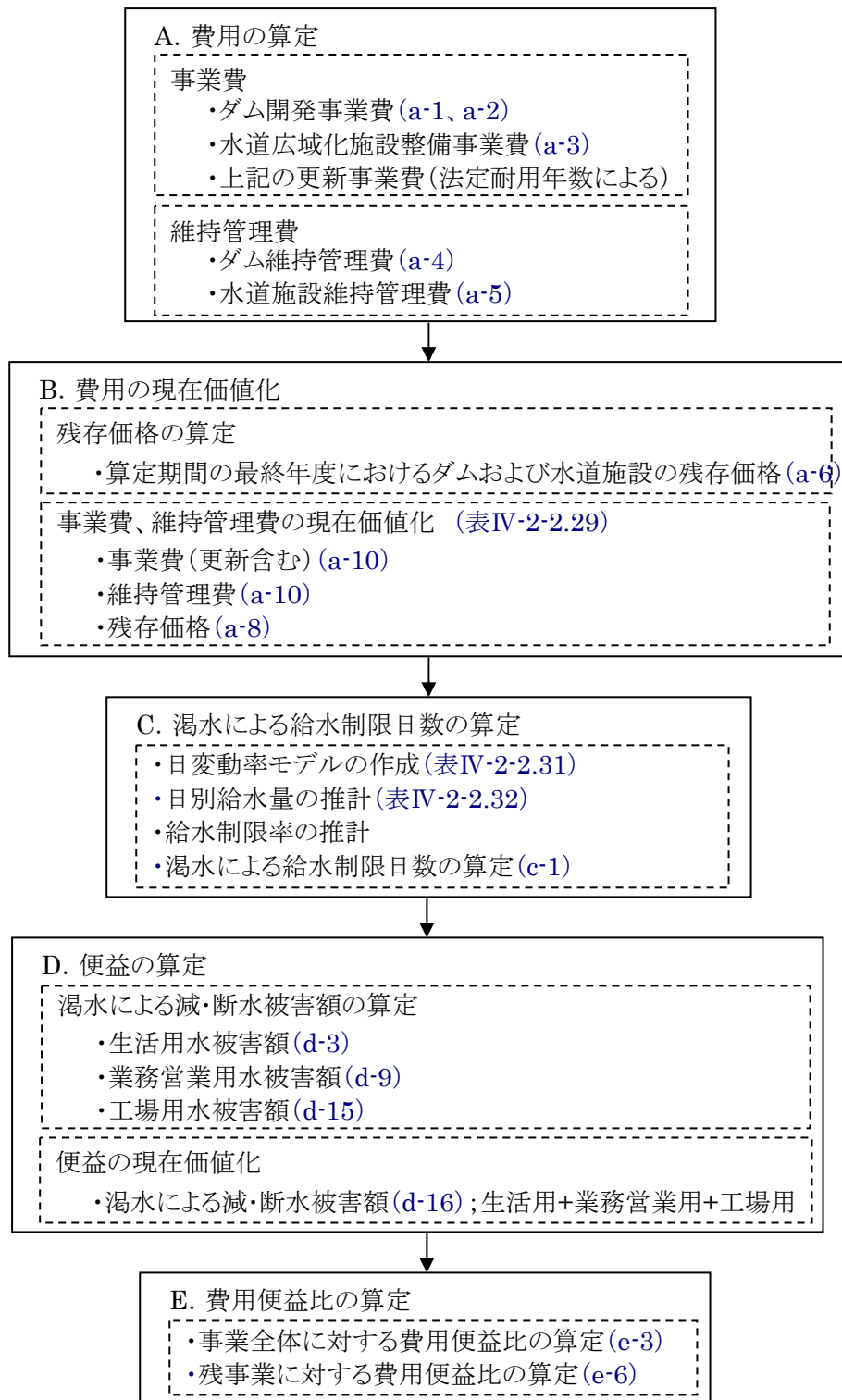
図Ⅳ-2-2.4 費用便益比の算定フロー
