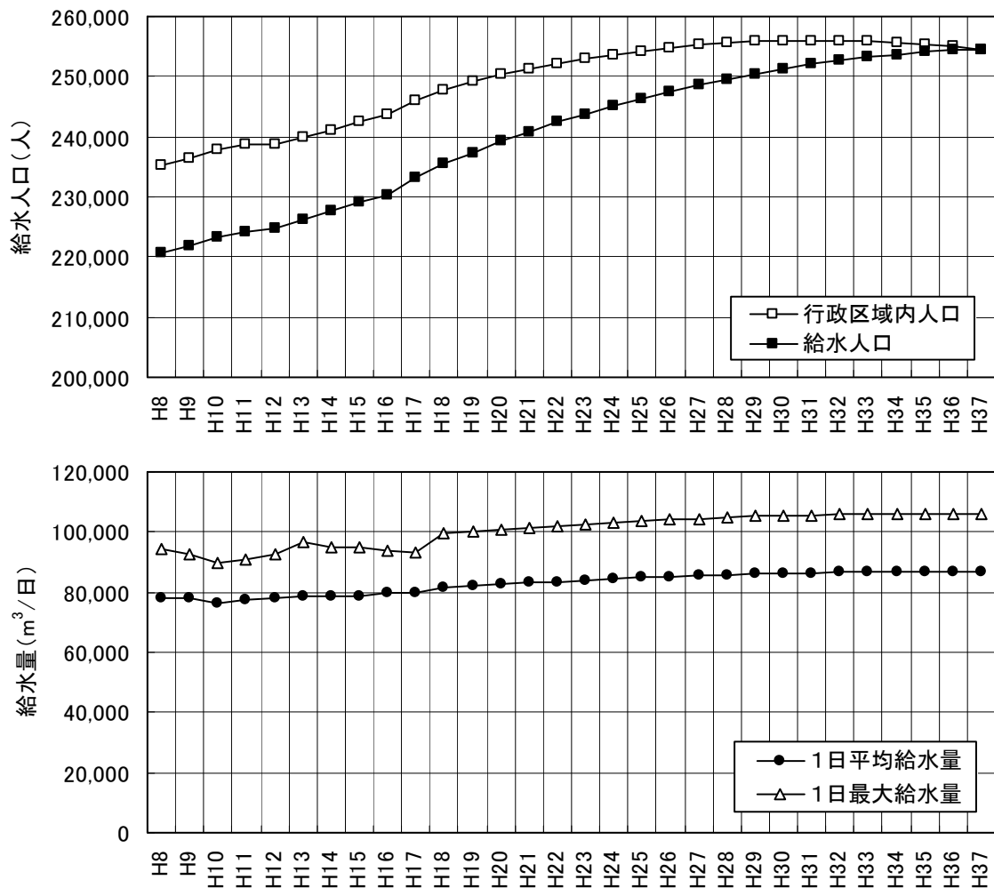
図Ⅳ-2-1.7 水需要予測
