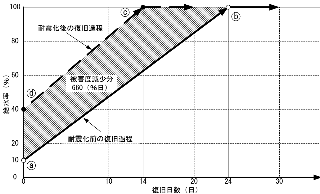
図Ⅳ-1-4.3 被害度減少分の算定
