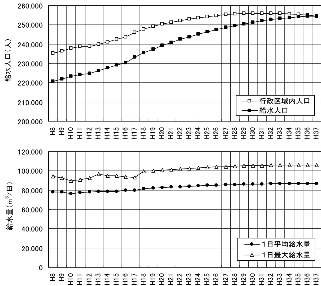
図Ⅳ-2-1.1 水需要予測
