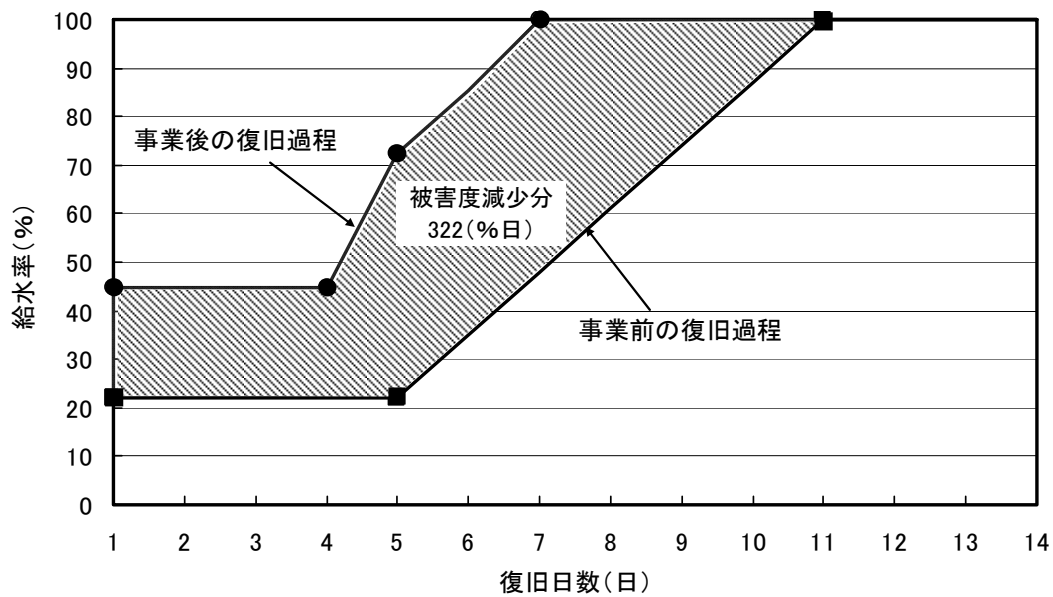
図Ⅳ-2-1.10 水質事故発生時の復旧過程
