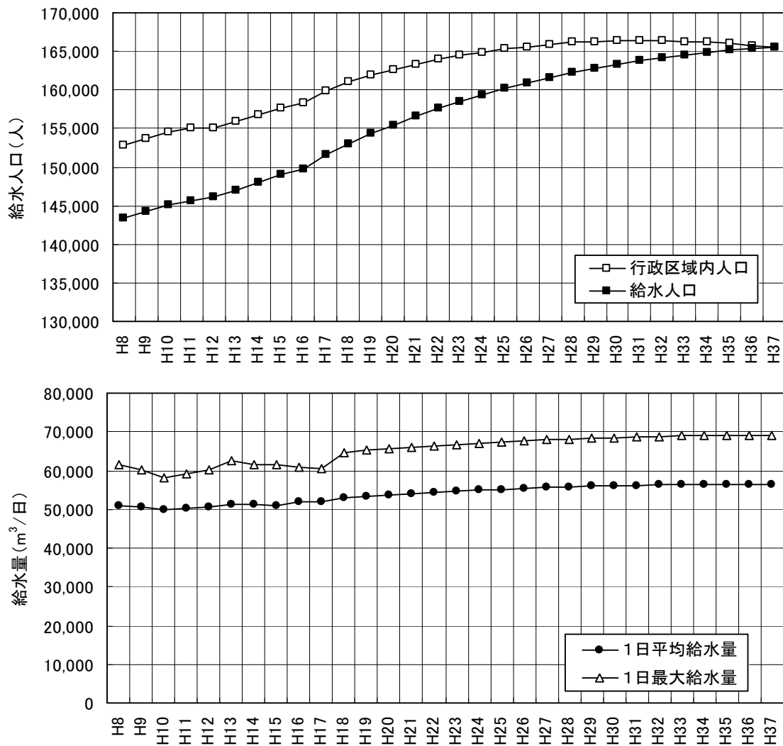
図Ⅳ-2-1.11 水需要予測
