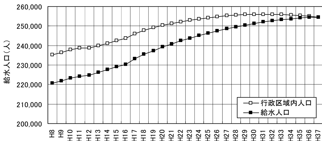
図Ⅳ-2-1.4 水需要予測(行政人口、給水人口)
