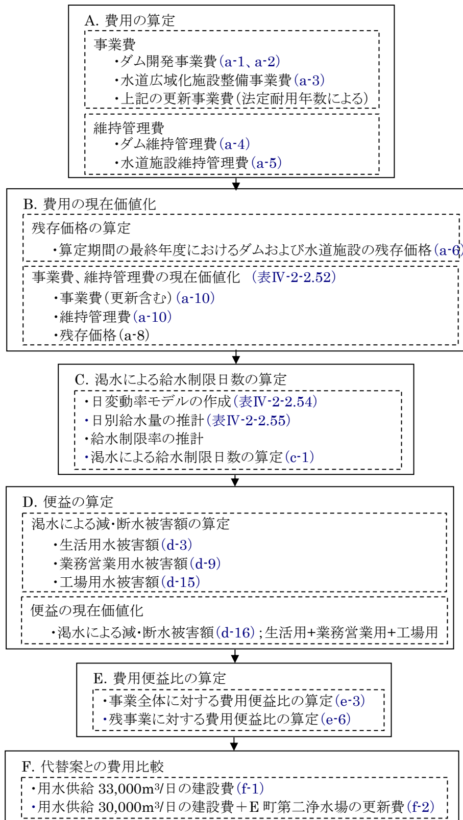
図Ⅳ-2-2.6 費用便益比の算定フロー
