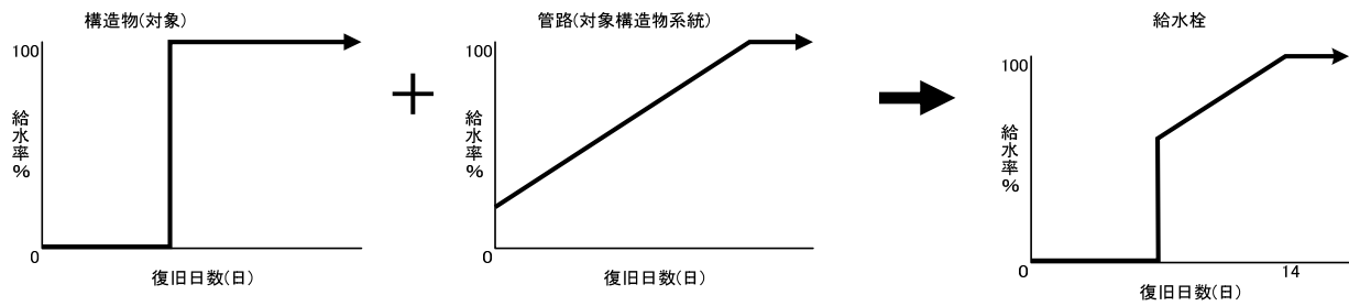
図Ⅳ-1-3.6 構造物を耐震化しない場合(without)の給水栓での被害のイメージ
