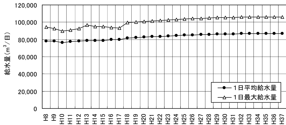
図Ⅳ-2-1.5 水需要予測(給水量)
