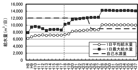
図Ⅳ-2.5 水需要予測(受水団体別)
