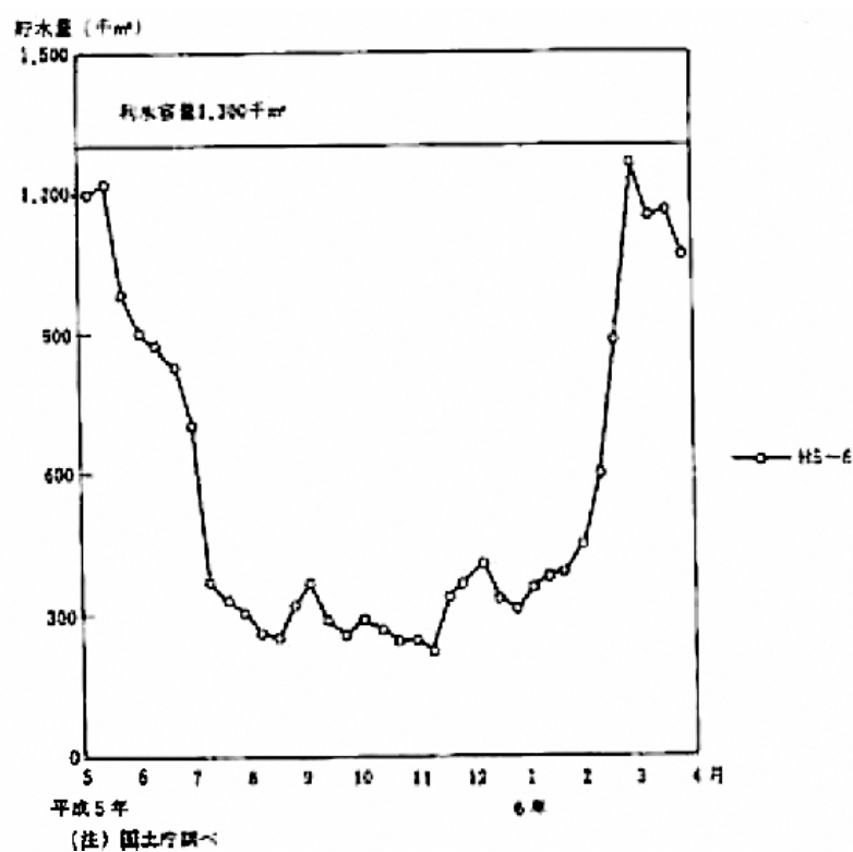
真栄里ダム貯水量図
