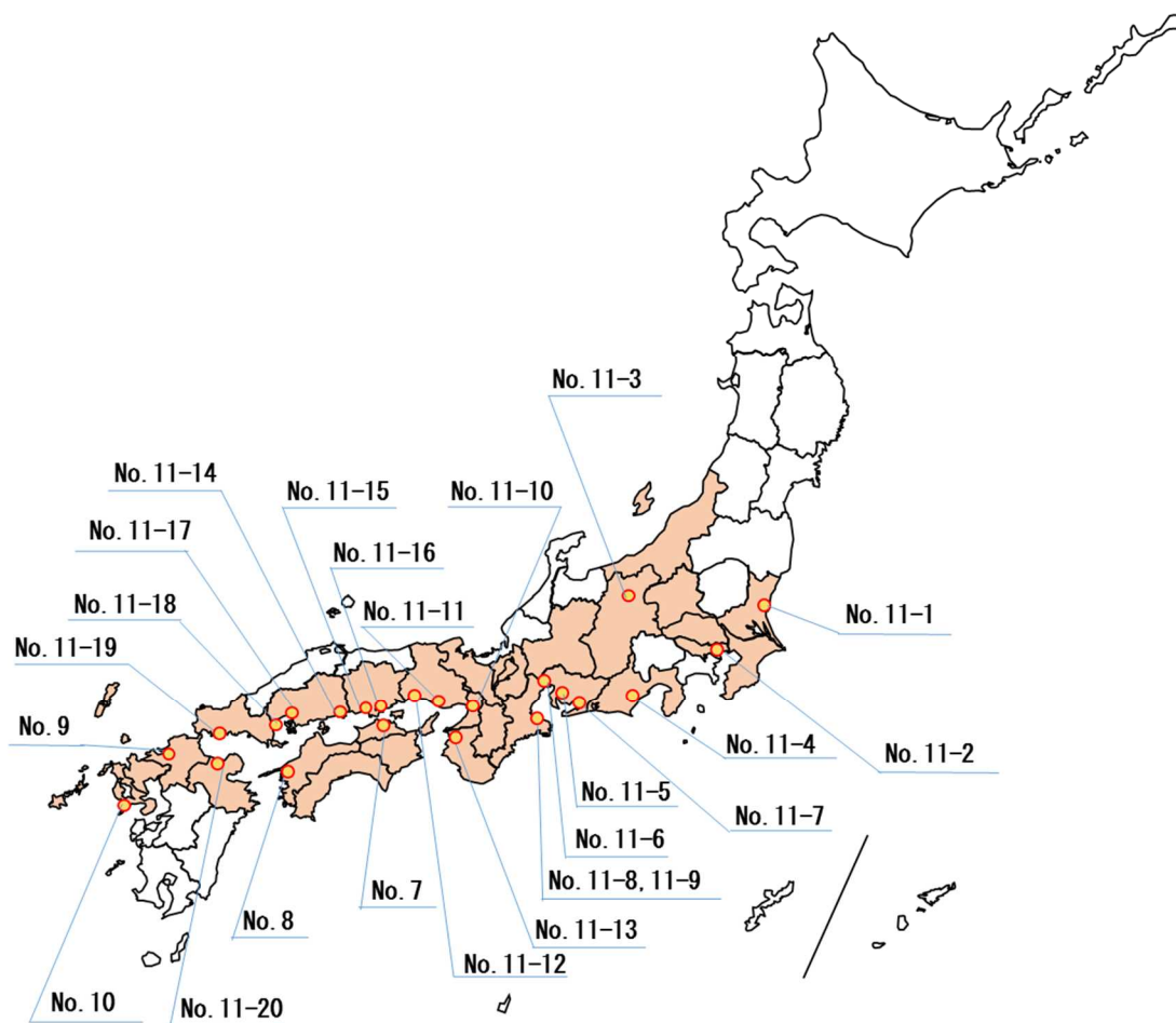
図 3.2 対象湧水の位置（平成6年列島湧水）
