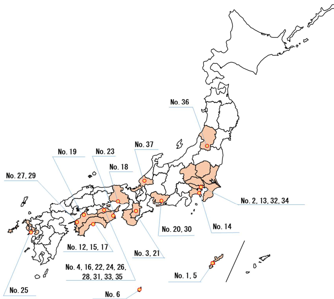
図 3.1 対象湯水の位置（平成 6 年列島湯水以外）
