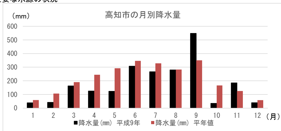
鏡川流域の月別降水量 (出典：過去の気象データ 気象庁HP)
