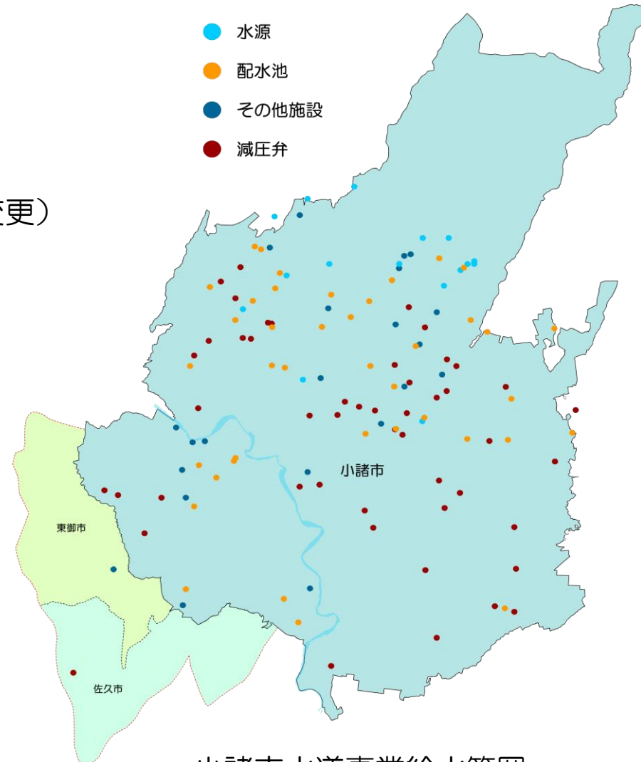
小諸市水道事業給水範囲
