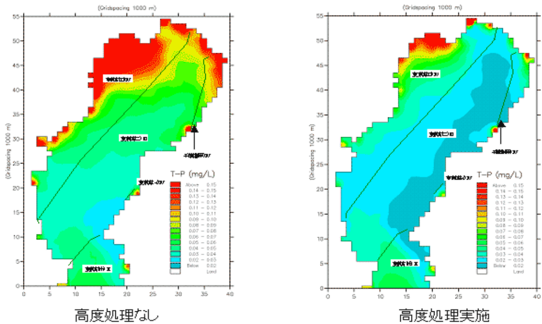
図3 - 4 高度処理の導入による東京湾の水質改善効果 (燐濃度)
