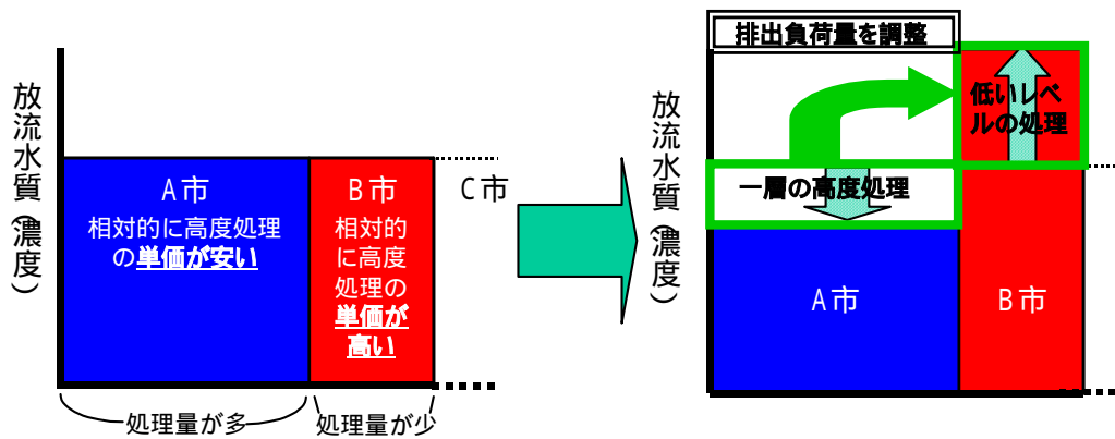
図3 - 5 排出負荷量調整の考え方
