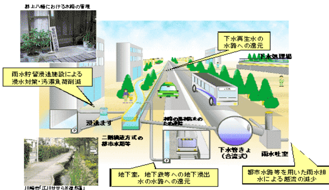
図6 - 1 水のネットワークと下水道との相互連携
