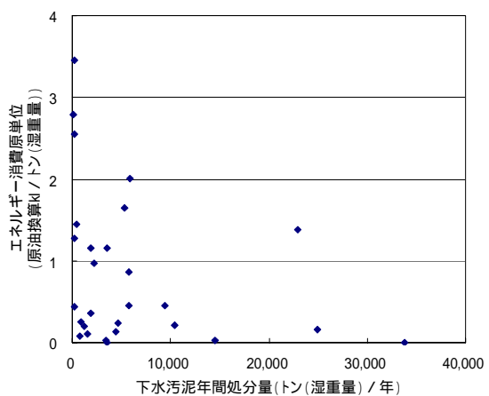
処理場のエネルギー消費原単位(汚泥処理のみ)
