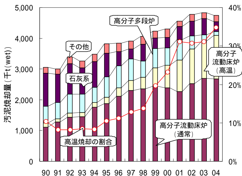
下水汚泥の焼却量の経年変化
