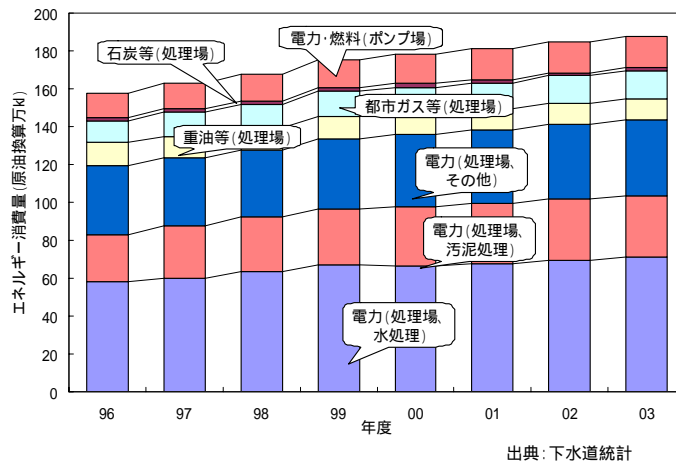
下水道施設のエネルギー消費量(一次エネルギー換算)
