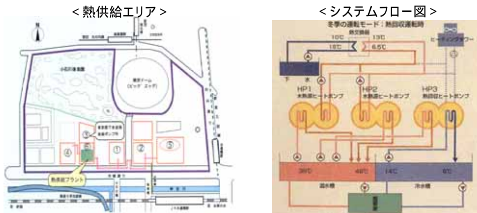
後楽ポンプ所の地域熱供給
