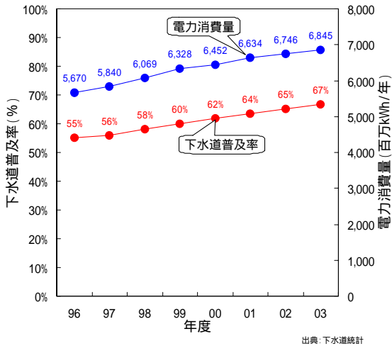
下水道施設の電力消費量の推移
