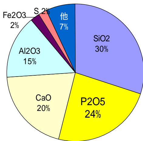
下水汚泥の無機分の組成
