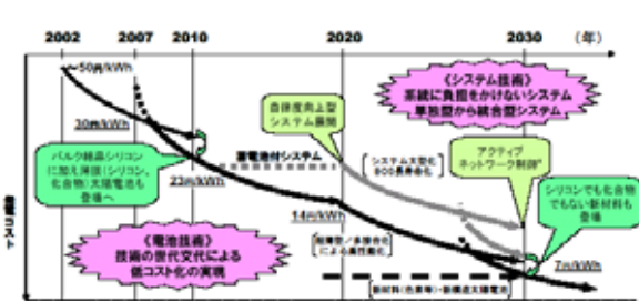
2030年に向けた太陽光発電の技術開発目標
