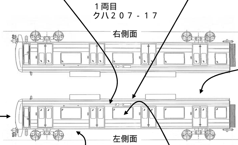
車体中間部の状況
