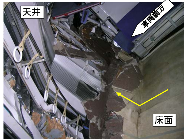
折れ曲がり部の状況（室内）
