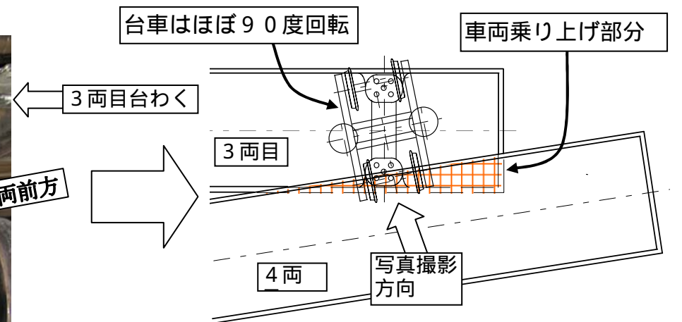
4 両目台わく 3 両目台わく 車両前方 後部台わく部の損傷状況 ( 4 両目が 3 両目に 乗り上げ )
