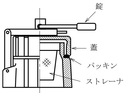
(b) 注油口金具
