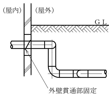
〔断面〕
