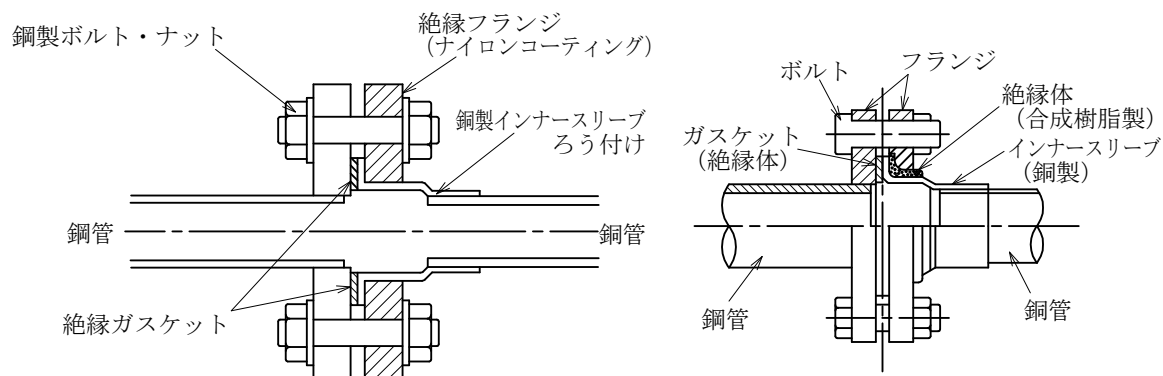
(1) 絶縁フランジの例
