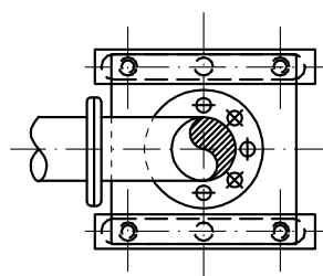
平面図
