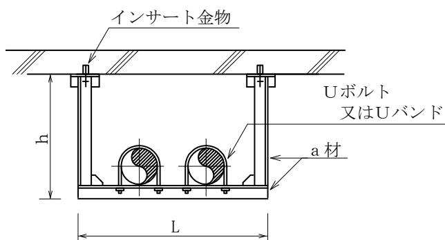
床の場合
