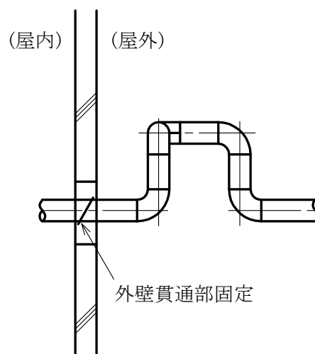
〔平面〕
