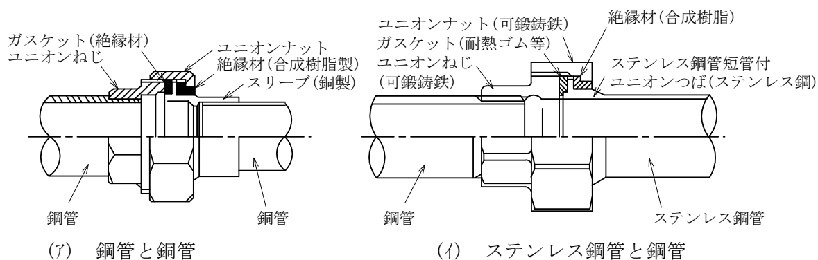
(4) 絶縁ユニオンの例
