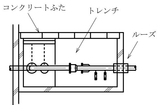
〔断面〕
