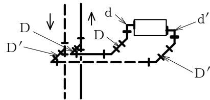
(b) 放熱器廻り(蒸気配管)
