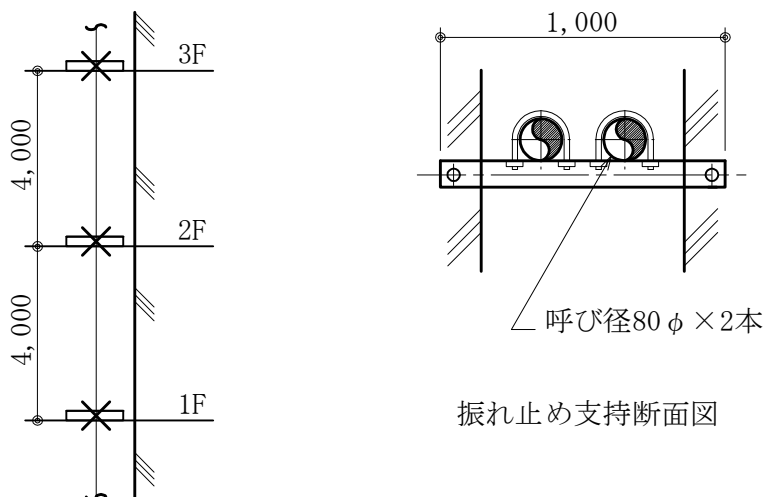
立面図 ×印部は振れ止め支持を示す。
