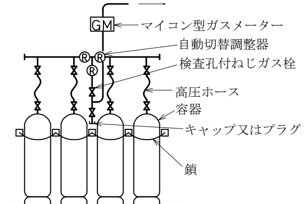
(b) 4本立て
