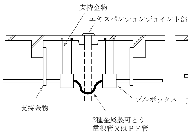
(断面)
