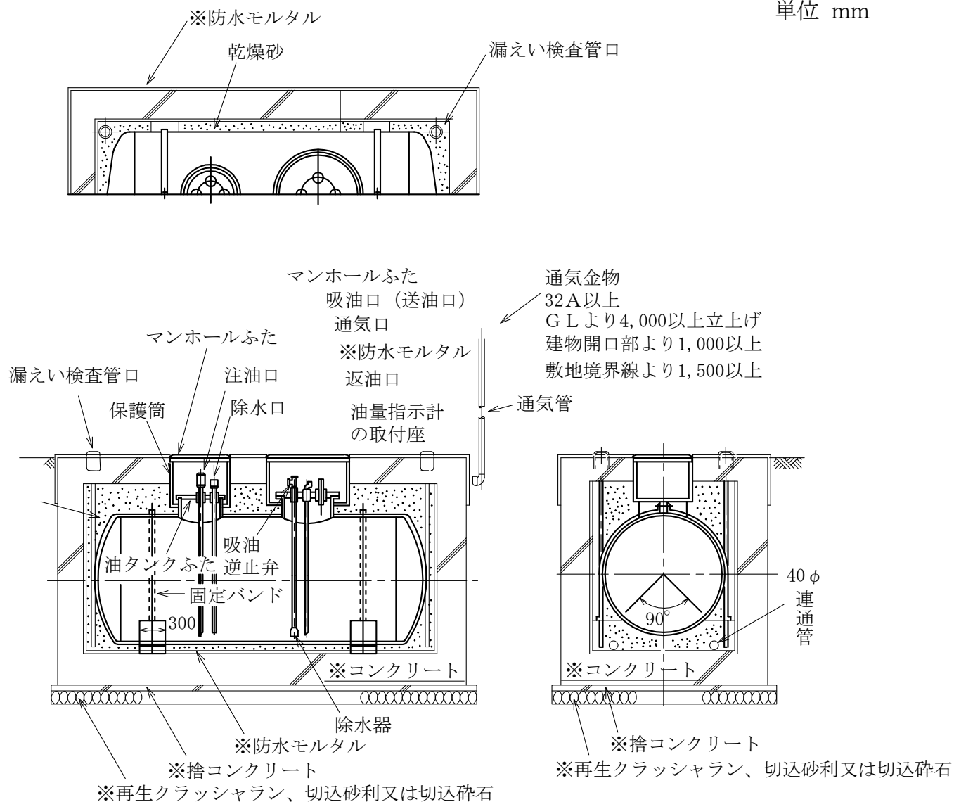
地下オイルタンク据付け図
