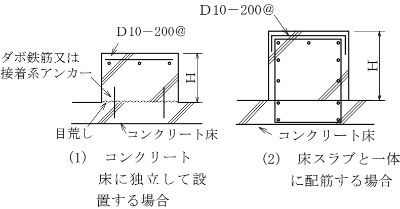
(a) 基礎の高さと配筋要領
