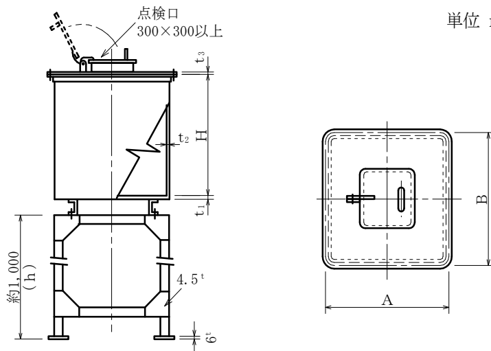
膨張タンク・消火用充水タンク TE・TF
