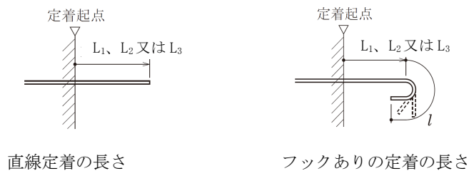
図 8.3.2 直線定着の長さ及びフックありの定着の長さ
