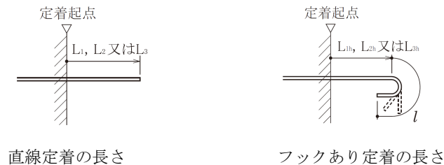
図 8.3.2 直線定着の長さ及びフックあり定着の長さ
