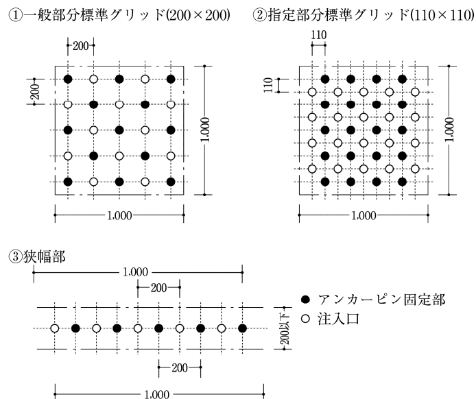
図 4.4.2 標準配置グリッド (mm)
