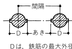
図 8.3.5 鉄筋相互のあき
