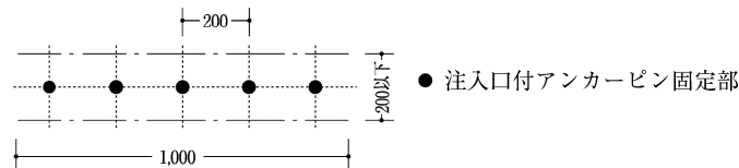
図 4.4.3 標準配置グリッド (mm)
