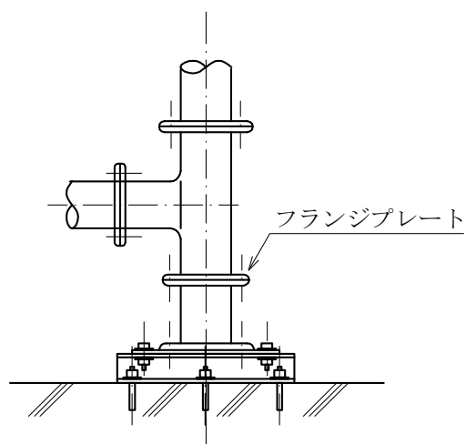
立面図
