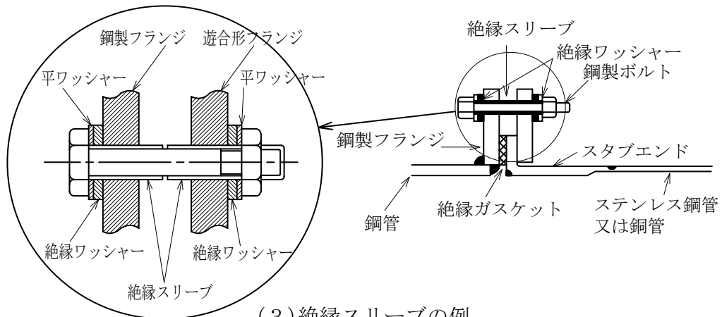
(3) 絶縁スリーブの例
