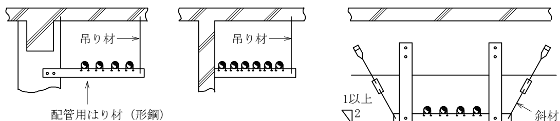
(4) 柱・壁等を利用する方法
