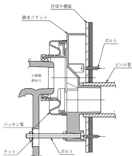
壁掛小便器
