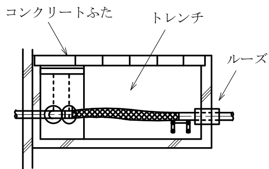
〔立面〕
