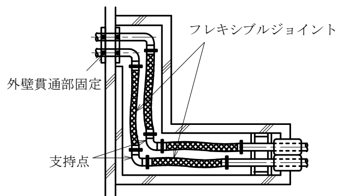
〔平面〕
