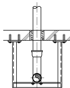
垂直部と曲り部
