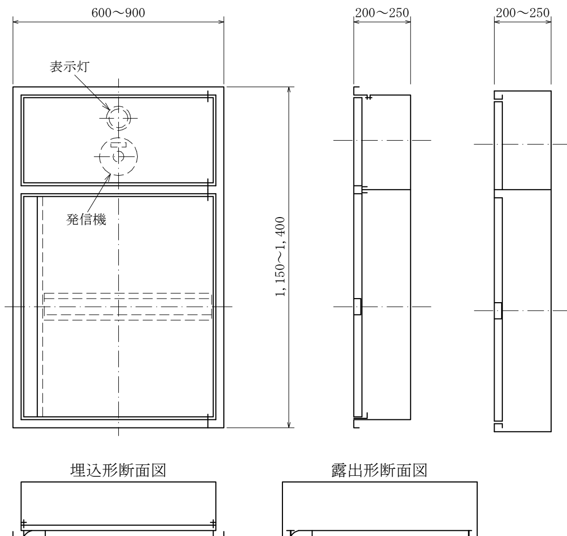
正面図
