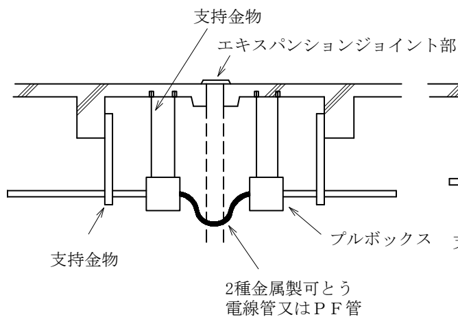
(断面)
