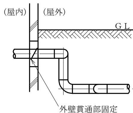
〔立面〕
