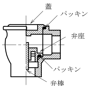
(a) 逆止弁
