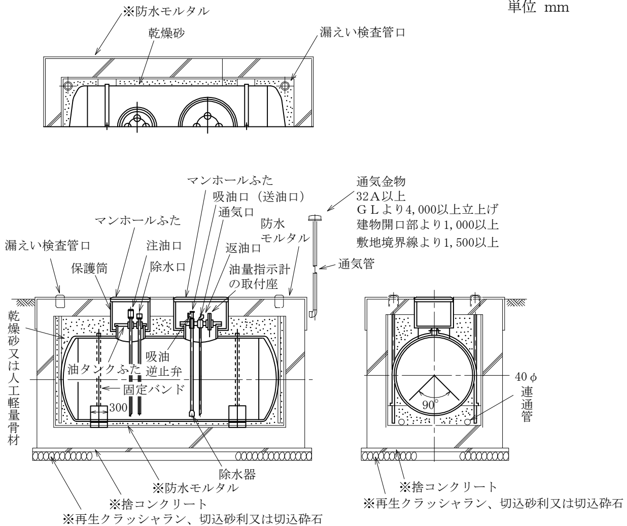
地下オイルタンク据付け図
