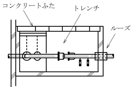
〔立面〕
