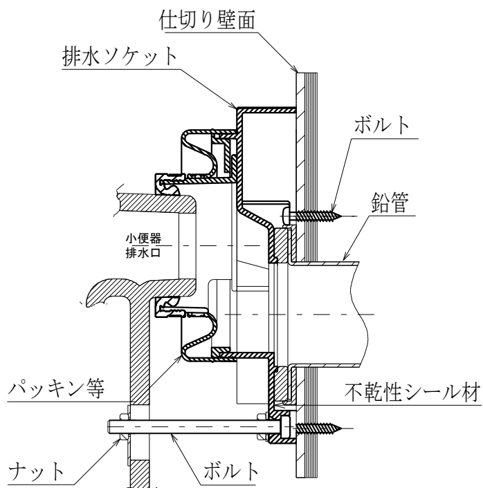
壁掛小便器
