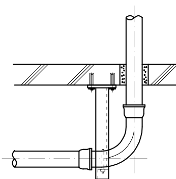
垂直部と曲り部
