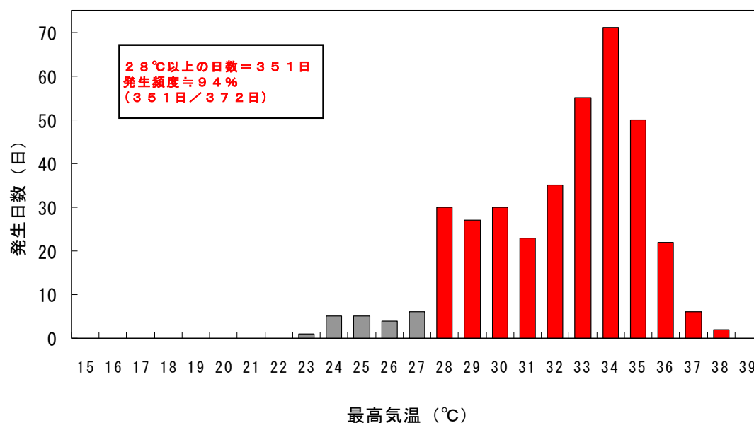
2002～2007 年の 7、8 月における大阪の日最高気温分布
