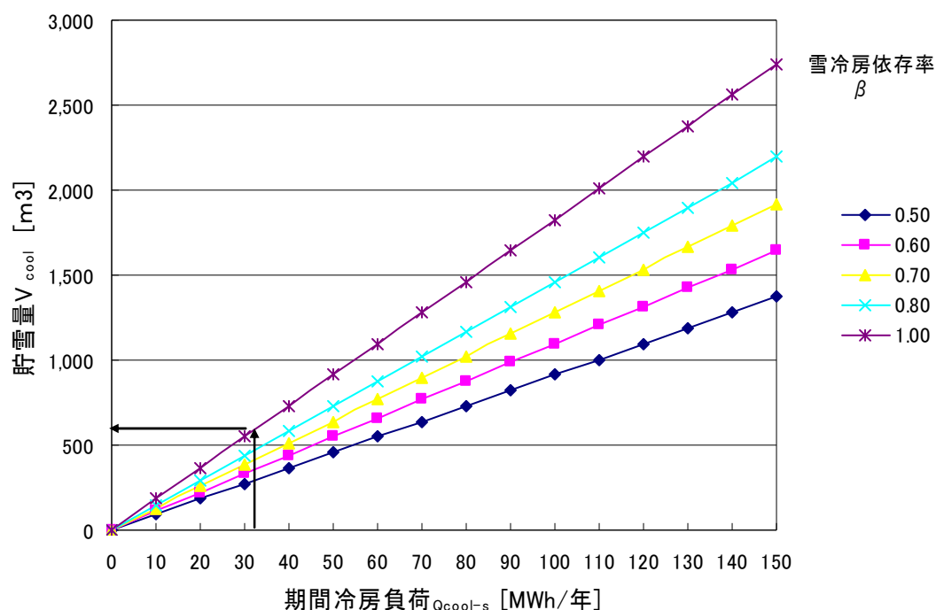
図 2-3 期間冷房負荷 Q_{cool-s} [kWh/年] に対する必要貯雪量 V_{cool} [m³/年]
