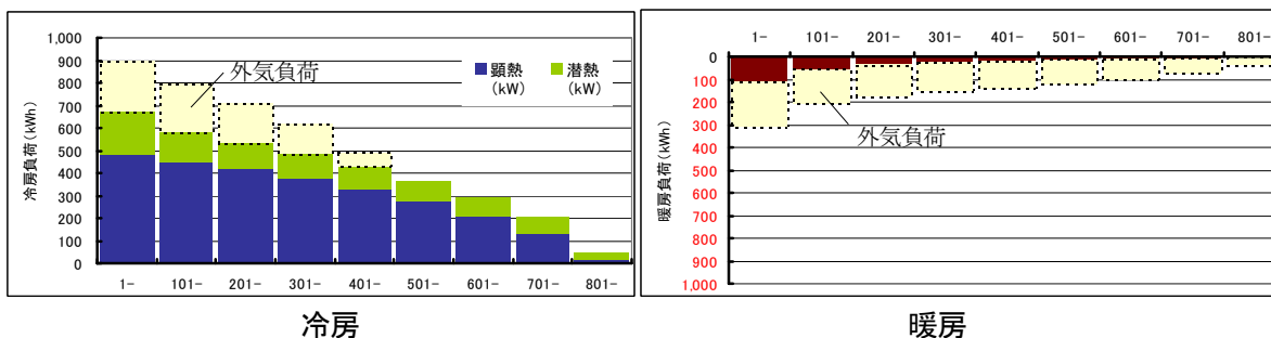
図2 熱負荷モード計算の境界条件（熱負荷<建物全体>）
