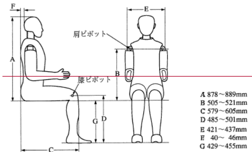
図 1 ハイブリッドⅢ構造寸法
