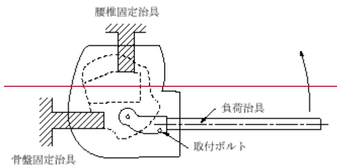
図9 大腿部の屈曲特性試験
