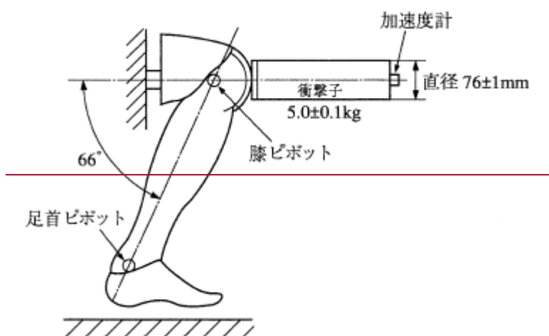
図8 脚部特性試験
