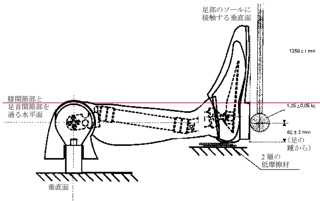
図 13—振り子衝撃子
