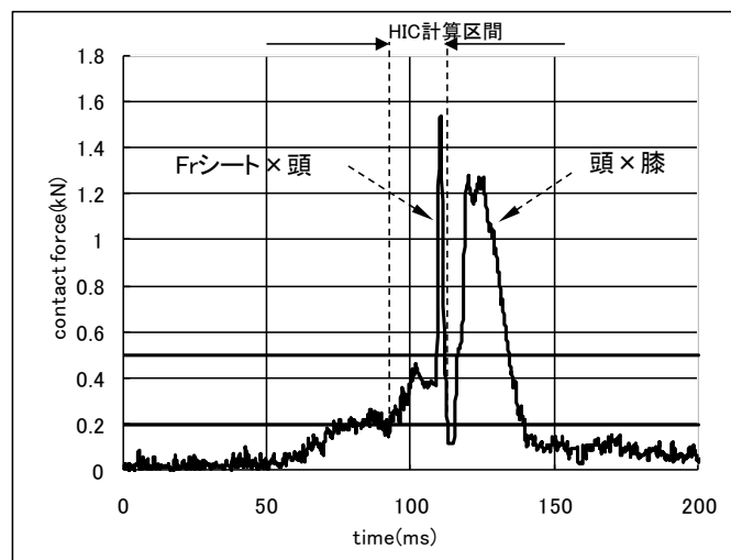
図5 接触荷重を分離でき、HIC 計算区間も分離可能な例
