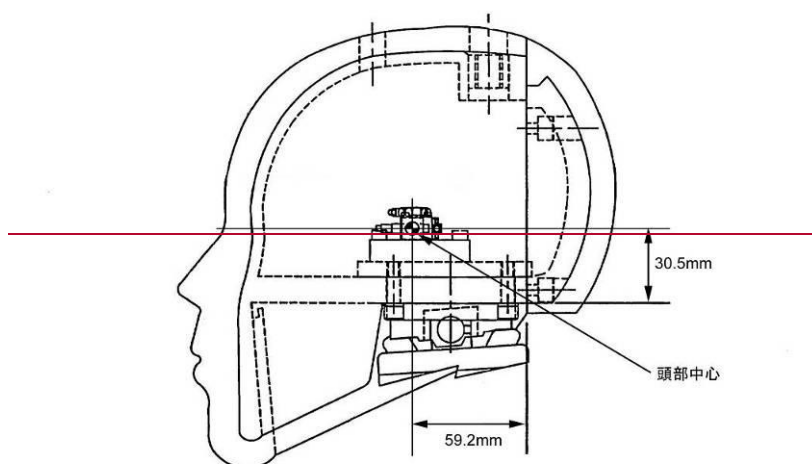
図 12 頭部加速度計感度中心
