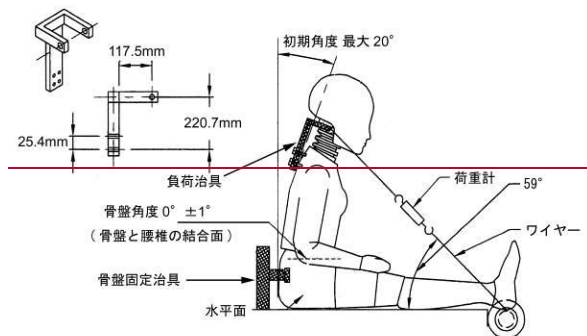
図 10 腰椎の屈曲特性試験
