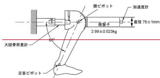
図 11 脚部特性試験
