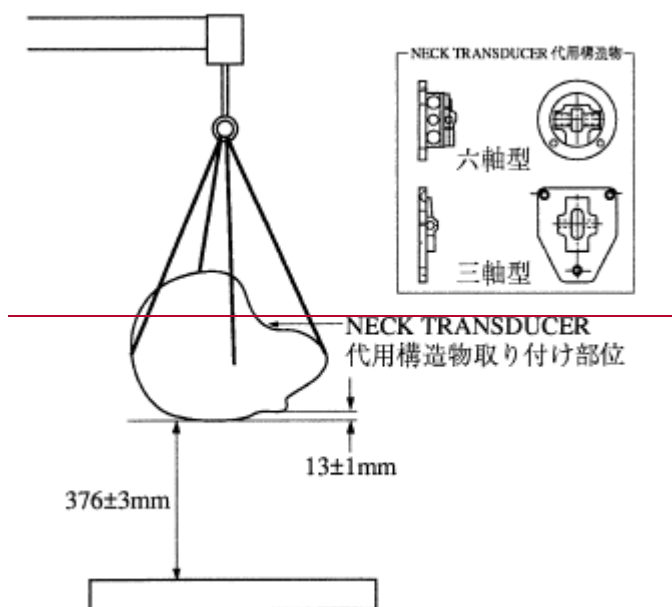
図2 頭部特性試験
