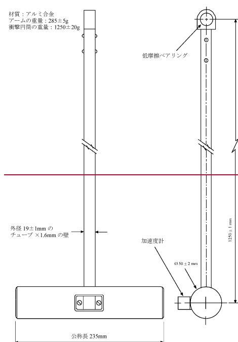
図 13—振り子衝撃子
