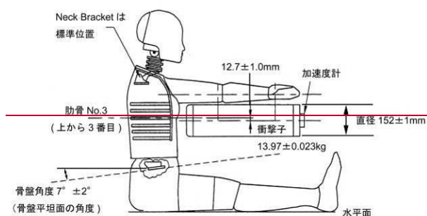
図8 胸部特性試験
