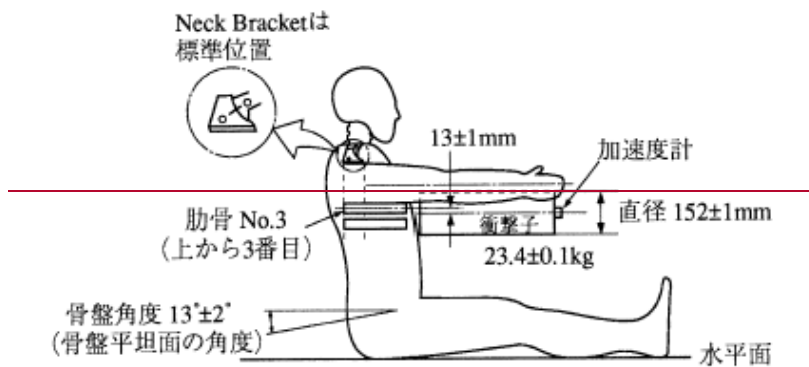
図 6 胸部特性試験
