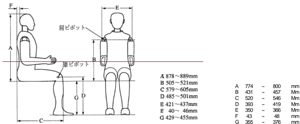
図 1 ハイブリッドⅢ構造寸法
