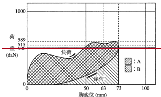
図 7 胸部特性試験荷重—変位曲線
