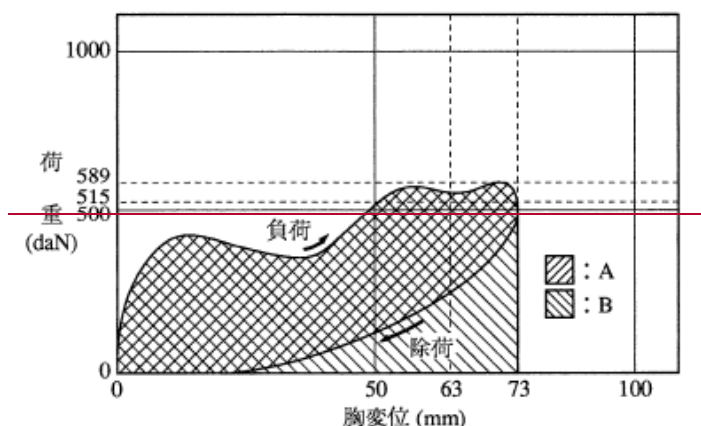
図 7 胸部特性試験荷重－変位曲線
