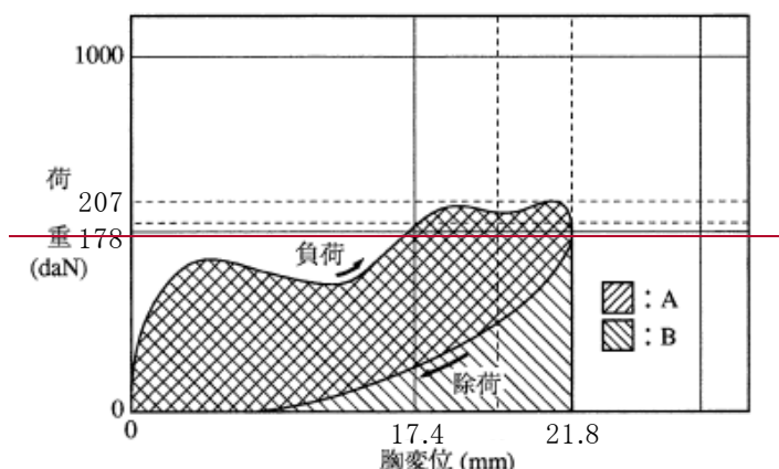
図9 胸部特性試験荷重—変位曲線
