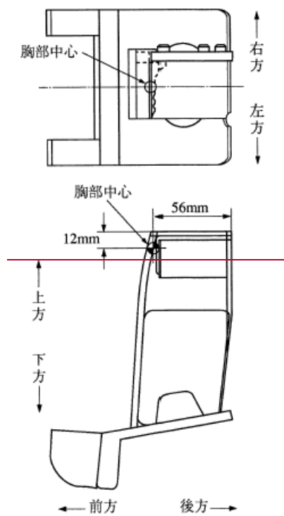
図17 胸部加速度計感度中心
