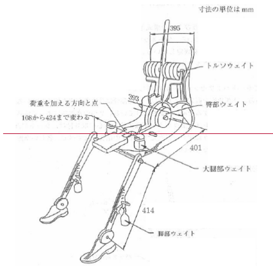
図2-3-DH測定装置の要素の寸法および荷重配分
