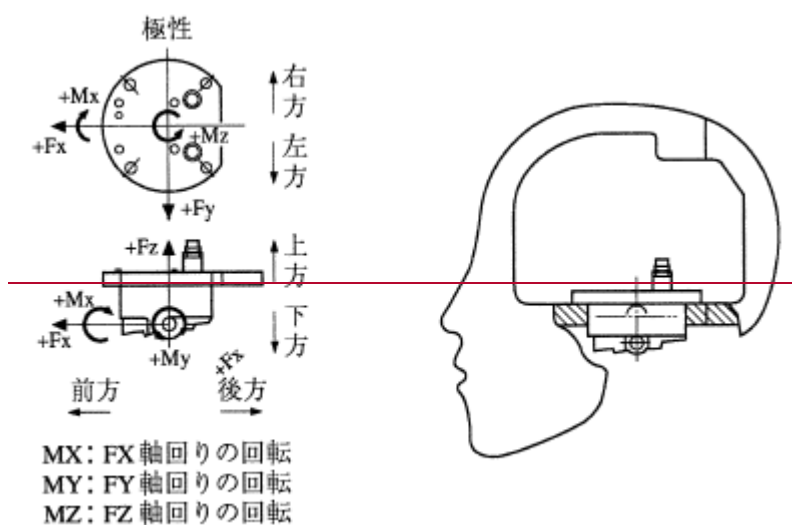
図 13 6 軸型首部荷重計取付状況
