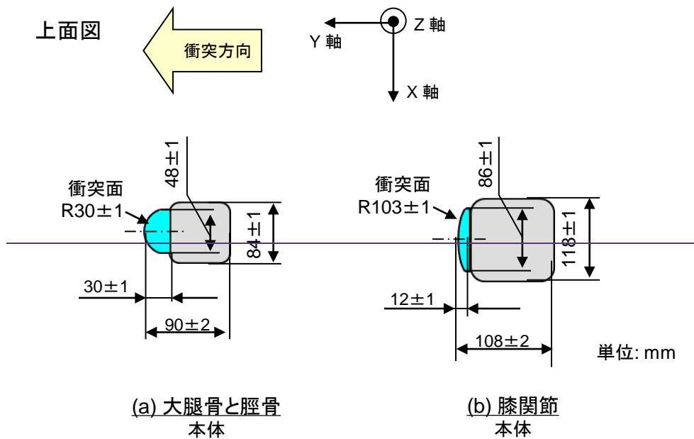
図1 脚部インパクト：大腿骨、膝部及び脛骨の寸法と重心位置（側面図）
