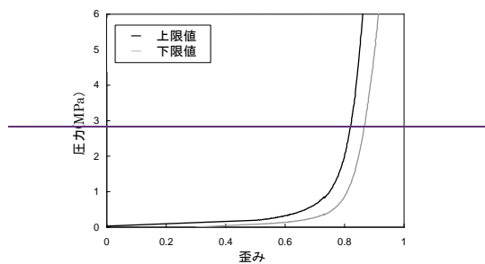
(b) ネオプレンシート
