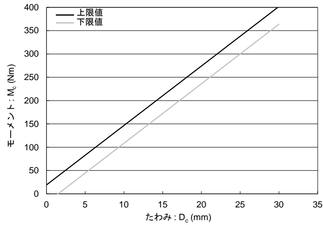
(b) 下腿骨曲げ変形コリド
