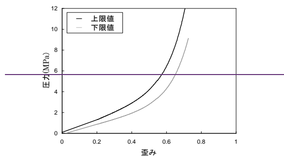
(a) 合成ゴムシート
