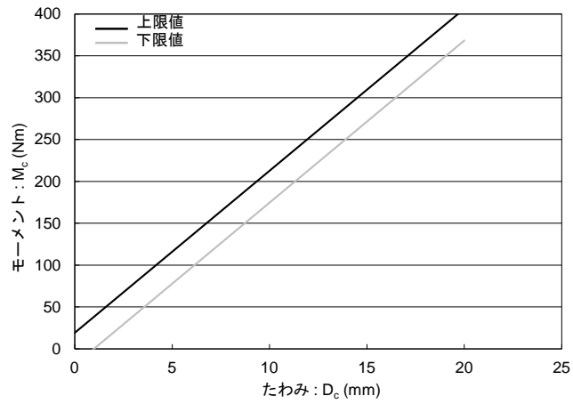
(a) 大腿骨曲げ変形コリド
