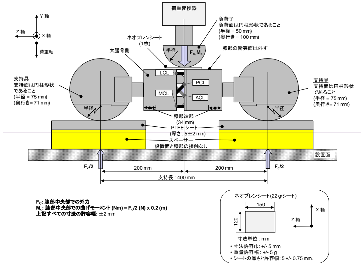
図10 膝部の静的検定試験セットアップ
