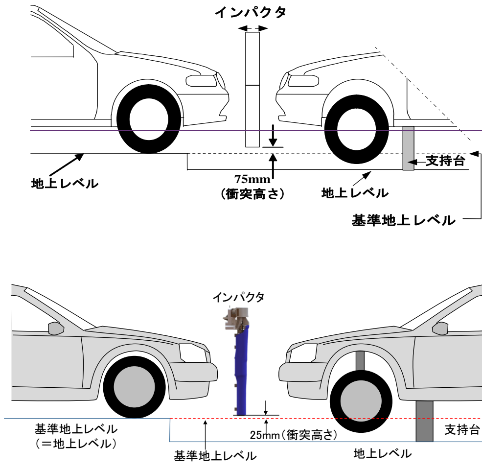
図 5.1 脚部インパクタの車両に対する初期衝突高さ (図左：完成車両、図右：支持台に載せた車両)
