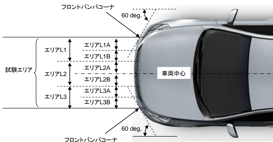
図 3.42 各試験エリアの呼称と分割
