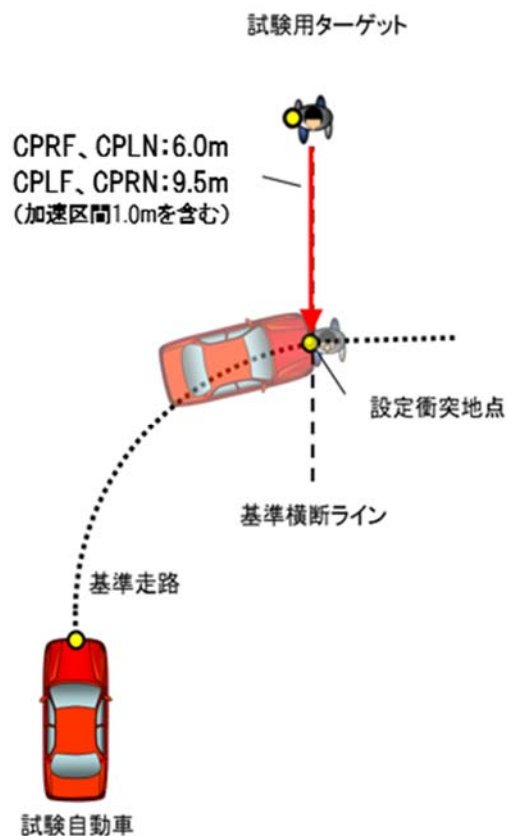
図 4 試験用ターゲットの初期位置
