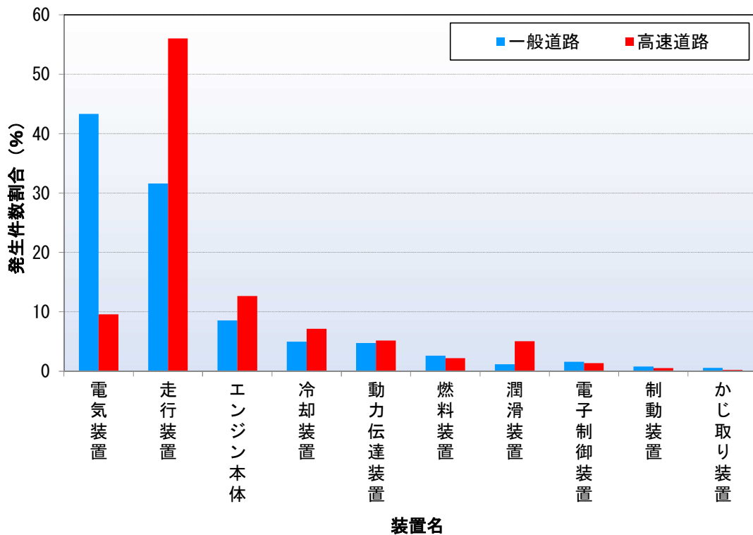
図1 道路別装置別故障発生件数の割合
