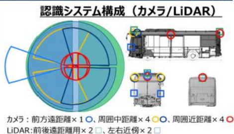
前後側方カメラ
