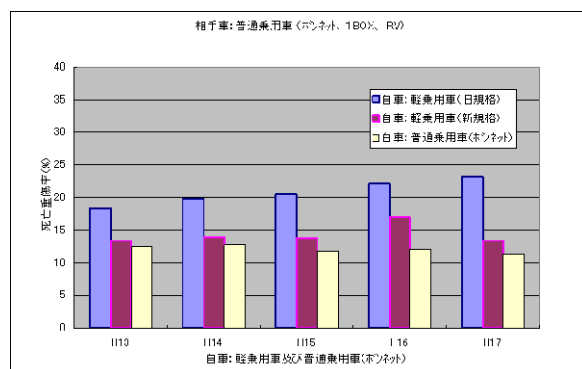
（図2）軽自動車のコンパチビリティ性能について
