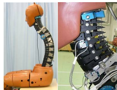
<BioRID ダミー>
