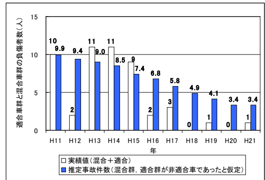
図 適合車群と適合・非適合混合群が仮に 対策されていなかった場合の年別負傷者数
