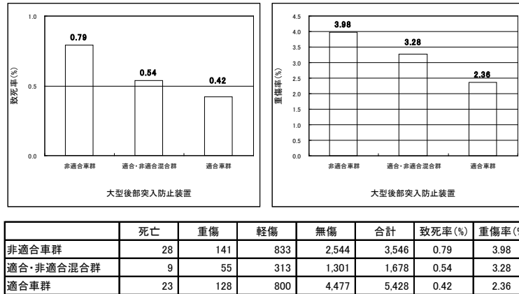
図 大型後部突入防止装置有無別の衝突相手車の致死率と重傷率
