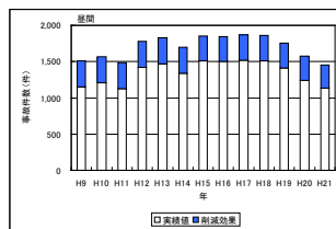
図 大型後部反射器がなかった場合の 推定事故件数 (注)
