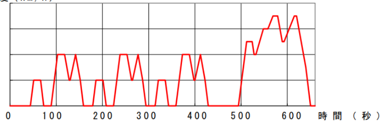
10・15モード
