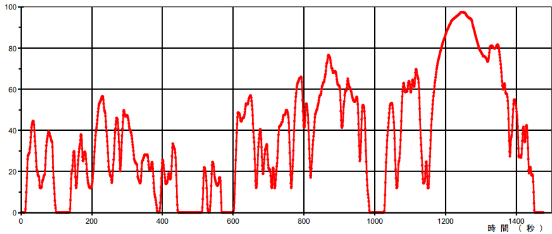
WLTCモード
