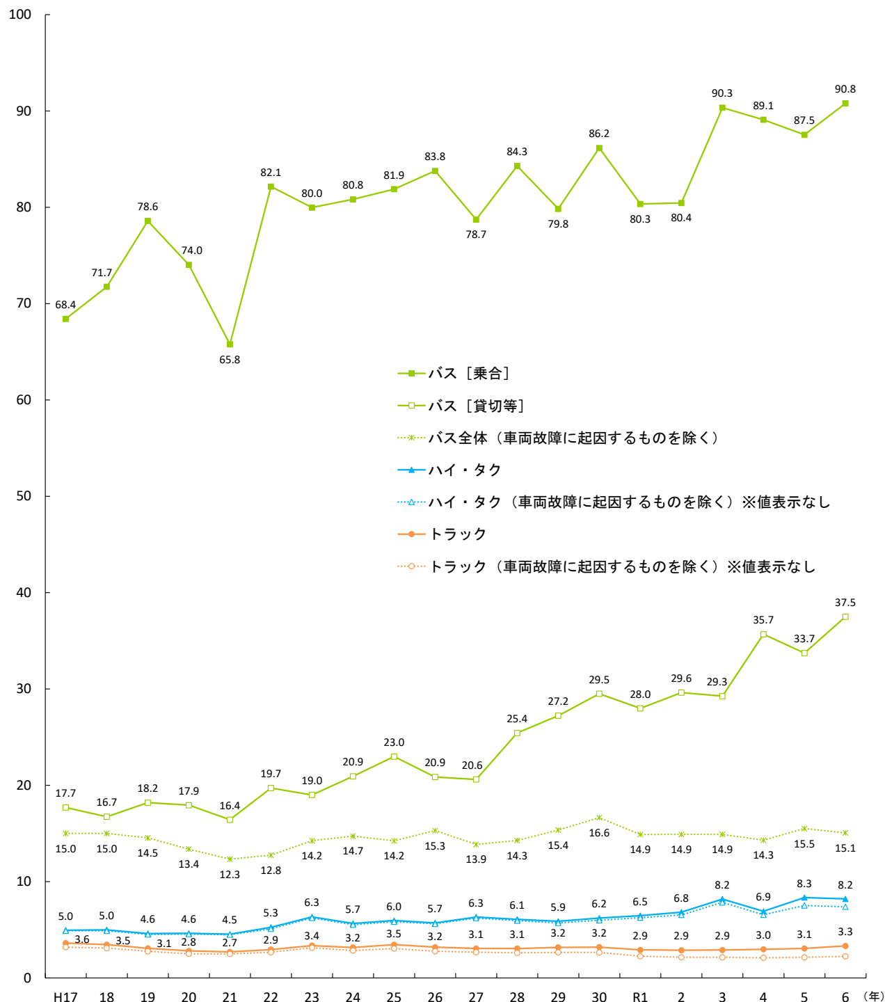
〔図2-4〕 業態別の事業用自動車1億走行キロ当たり重大事故件数の推移
