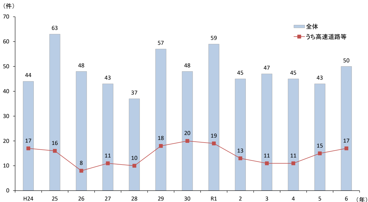
〔図6-1〕 危険物等積載運搬車両の重大事故発生状況の推移
