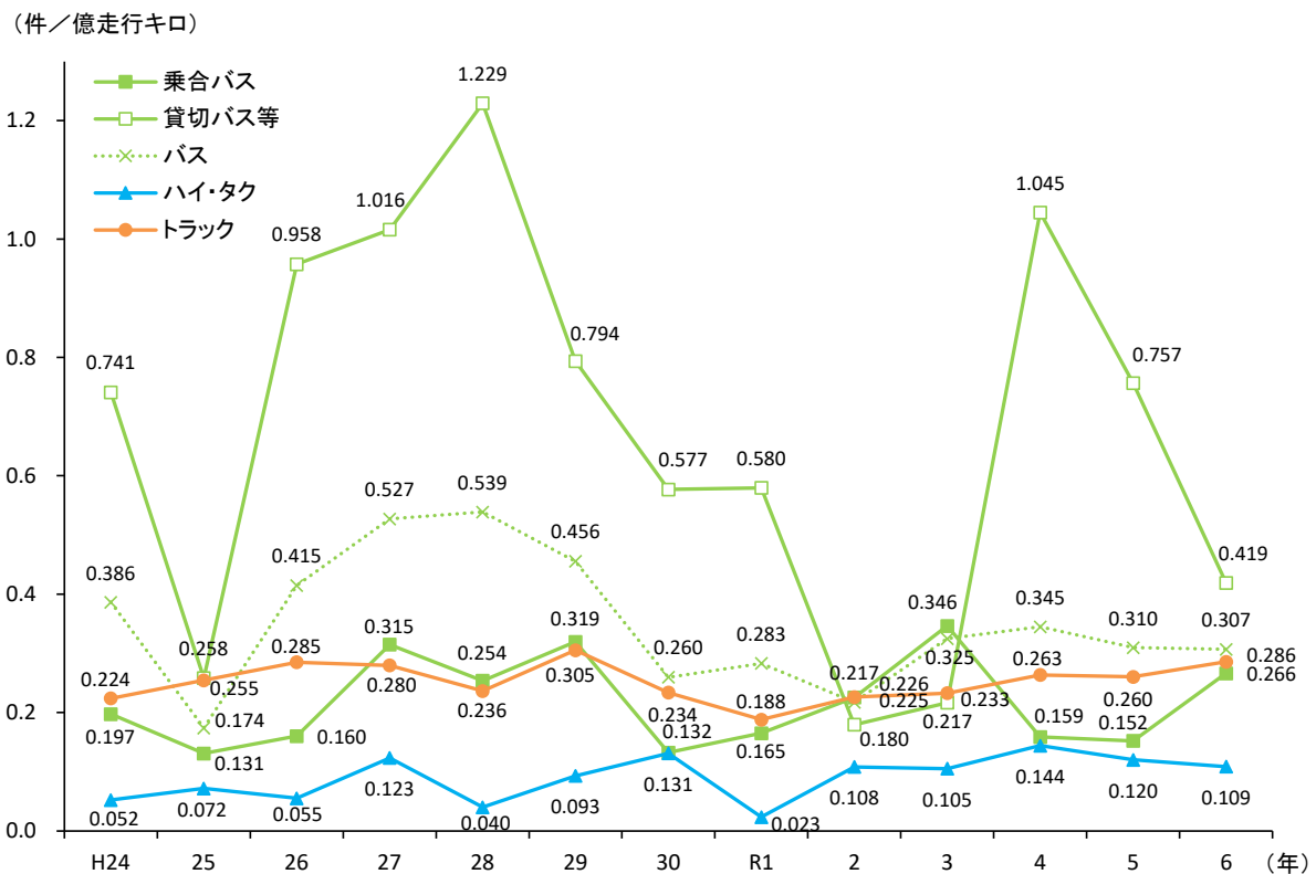
〔図5-2〕 業態別の事業用自動車1億走行キロ当たり火災事故発生件数の推移
