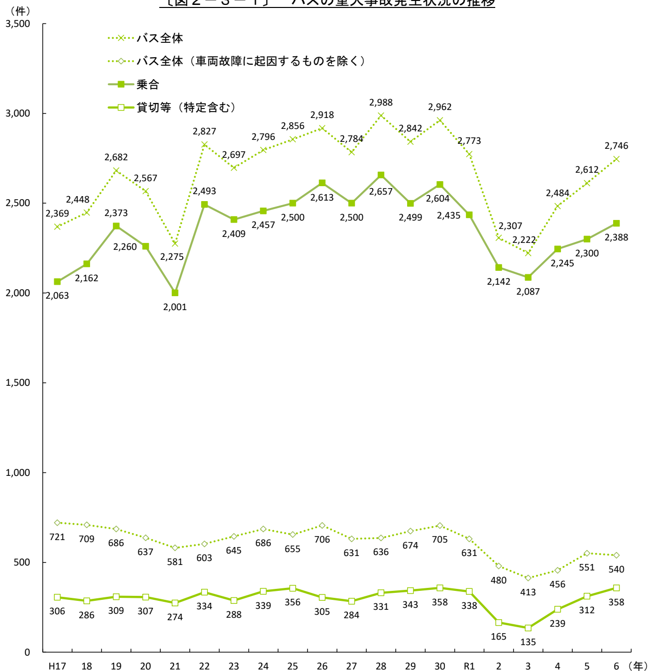
〔図2-3-1〕 バスの重大事故発生状況の推移
