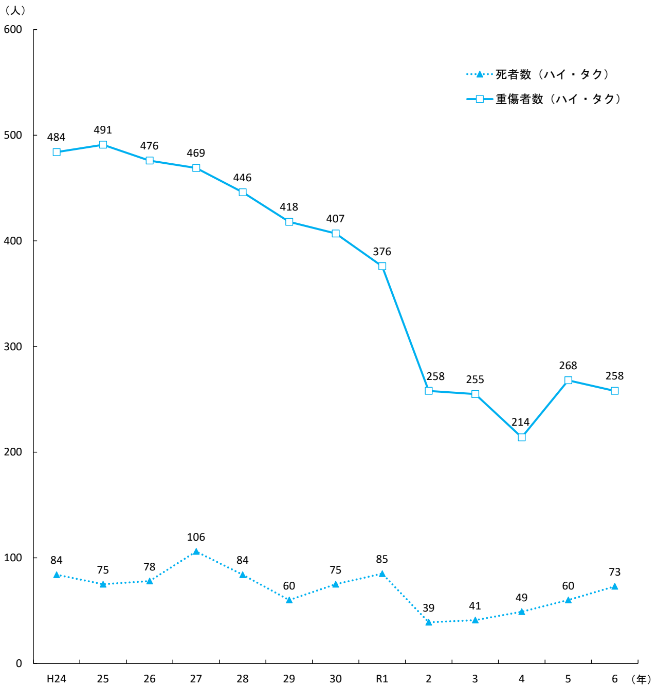
[図 2-5-2 (2)] タクシーの重大事故による死者数及び重傷者数の推移 (車両故障に起因するものを除いた重大事故)
