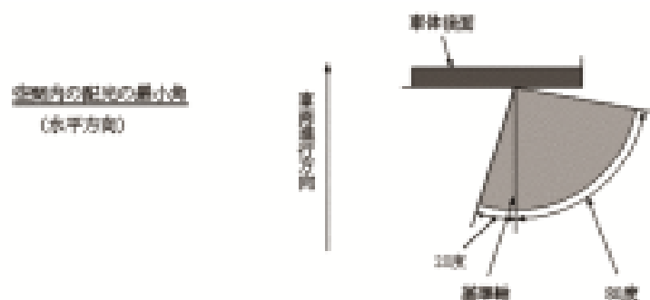
図2 尾灯のH面の高さが地上750mm未満となるように取り付けられている場合の当該尾灯のH面より下方の最小角：
