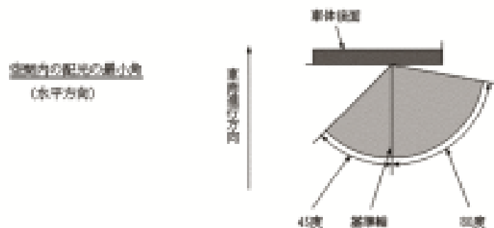
図1 尾灯のH面の高さが地上750mm以上となるように取り付けられている場合の当該尾灯のH面より下方の最小角：
