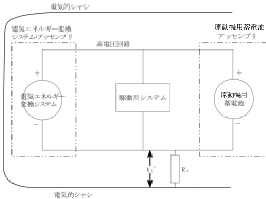
図2 V'_i の測定
