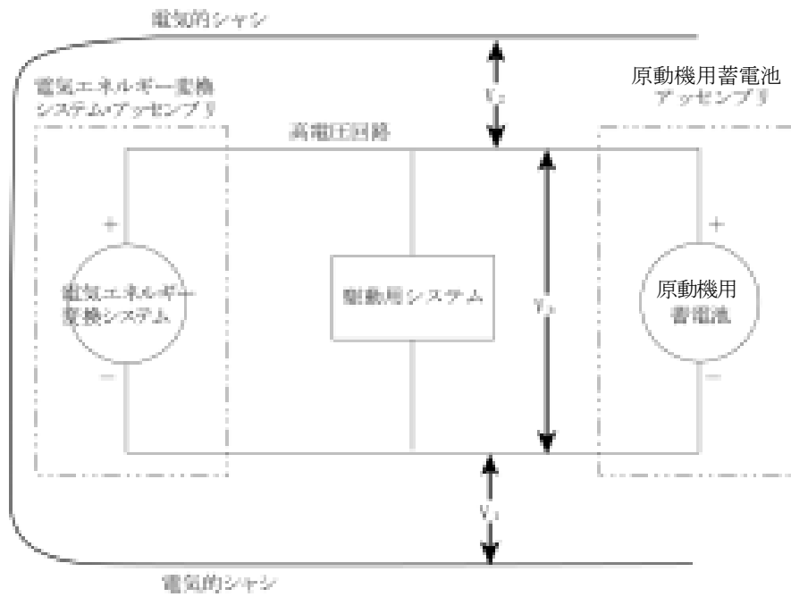
図1 V_b 、 V_i 及び V_2 の測定
