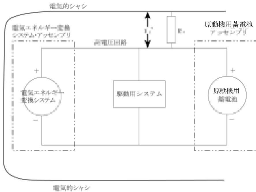
図3 V_2' の測定
