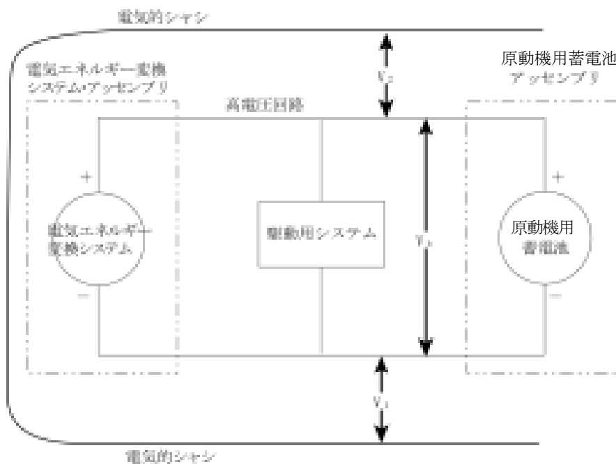
図 V_b 、 V_1 及び V_2 の測定
