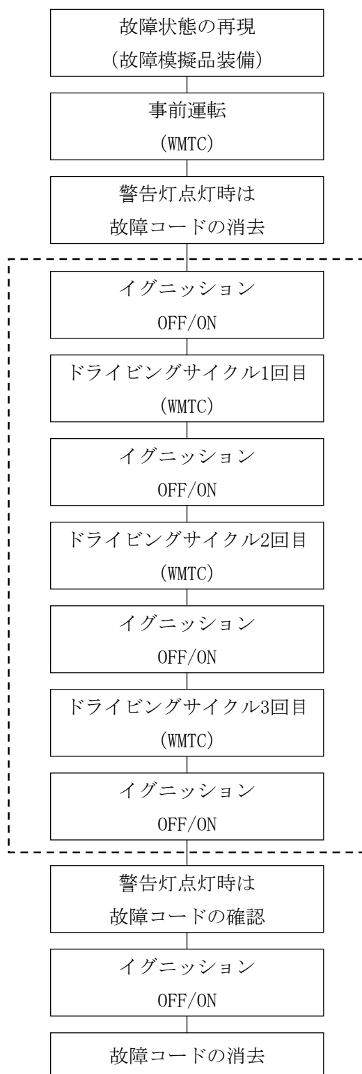
図1 故障検知の基準適合性の確認方法手順（例）
