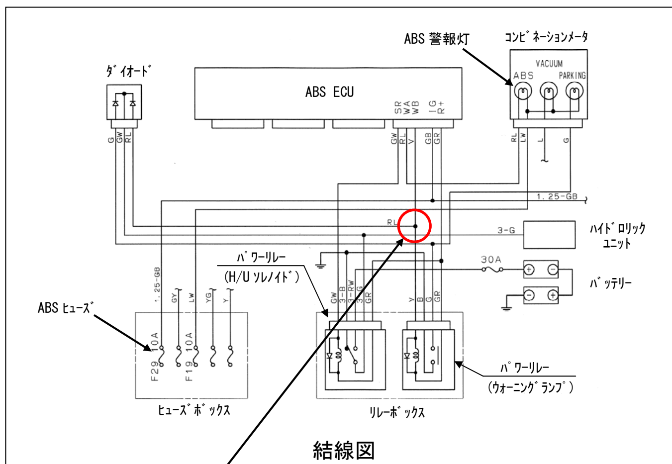
実体配線図
