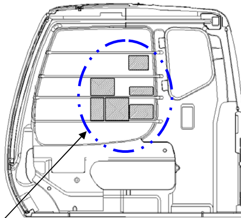
運転室断面図
