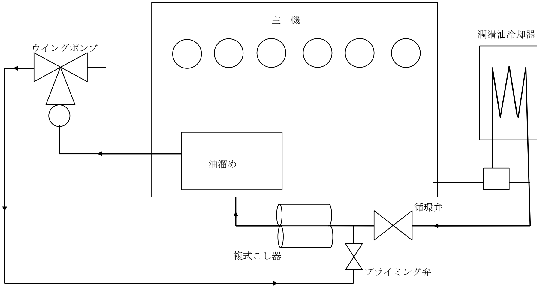
潤滑油系統略図
