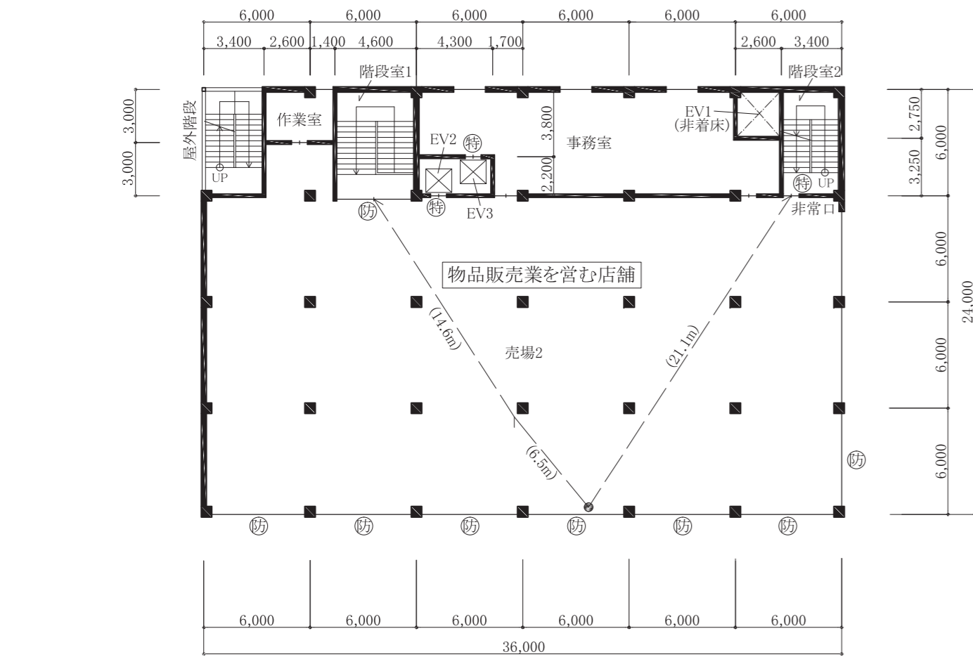
2階平面図
