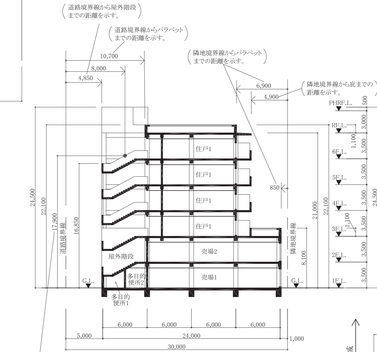
A-A'断面図
