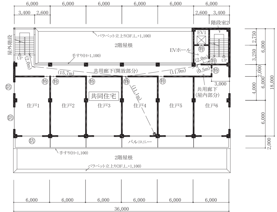
3~6階平面図
