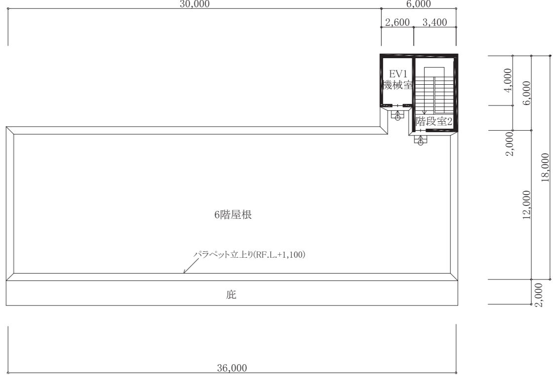
屋上階平面図
