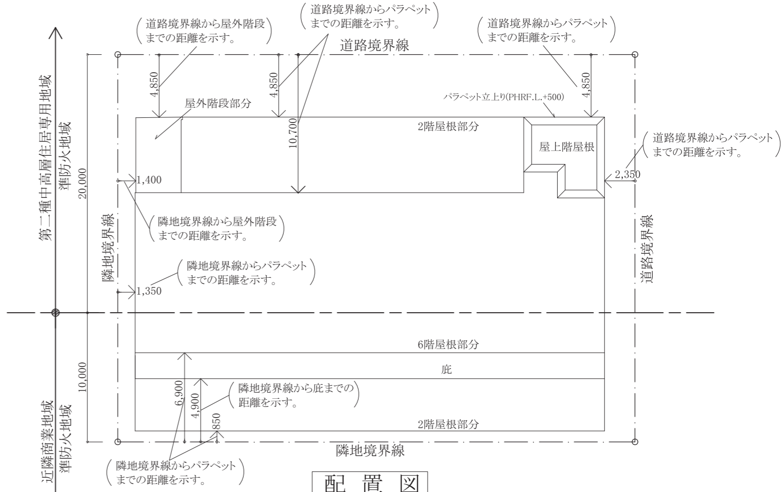
配置図
