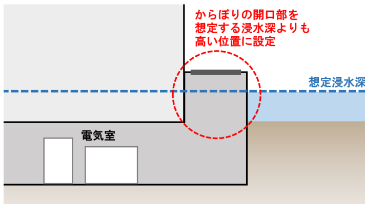
図：からぼりの嵩上げのイメージ (地下の電気室につながるマシンハッチの例)
