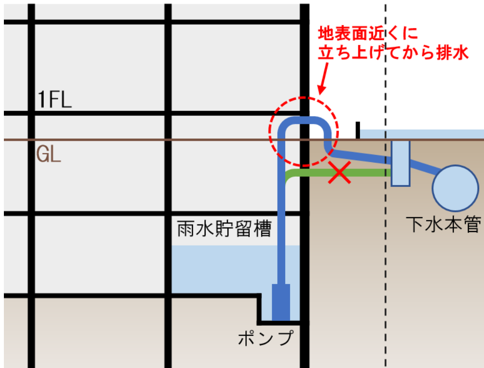
図：排水設備の配管における立上り部の設置イメージ
