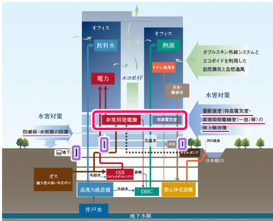
図：BCP機能説明図
