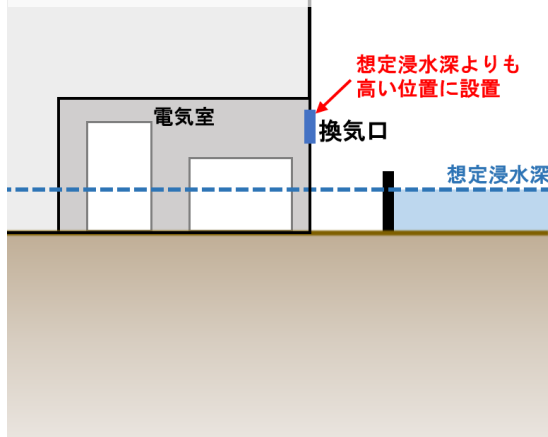
図：換気口の位置の工夫のイメージ
