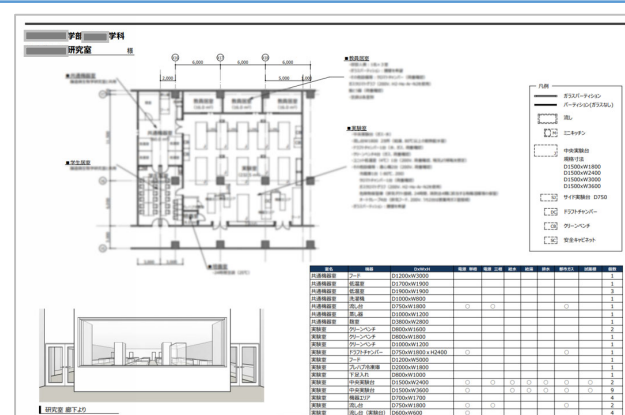
BIMを活用したヒアリング手法により作成したレイアウトプラン
