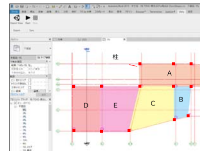
構造設計モデル
