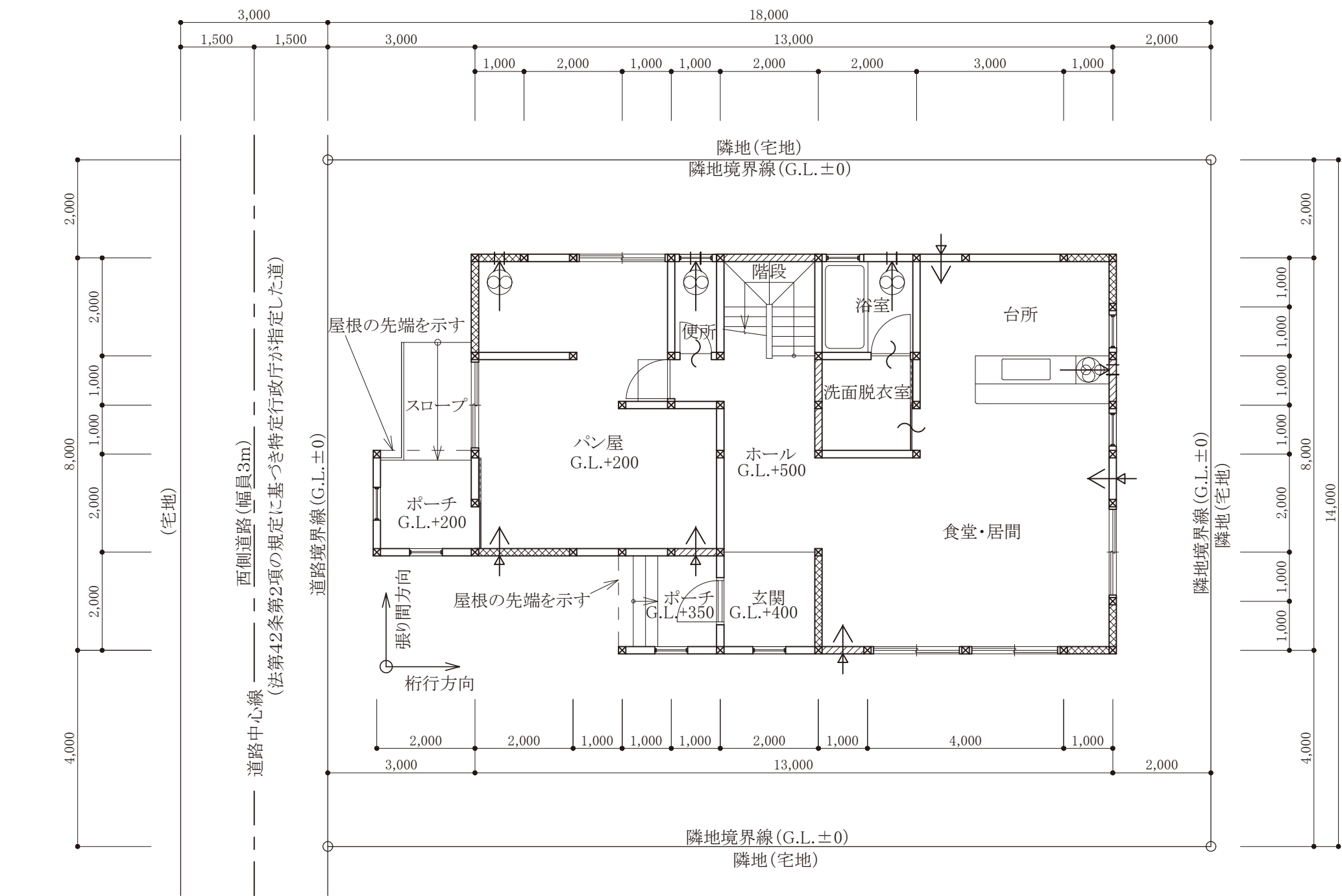
1階平面図・配置図
