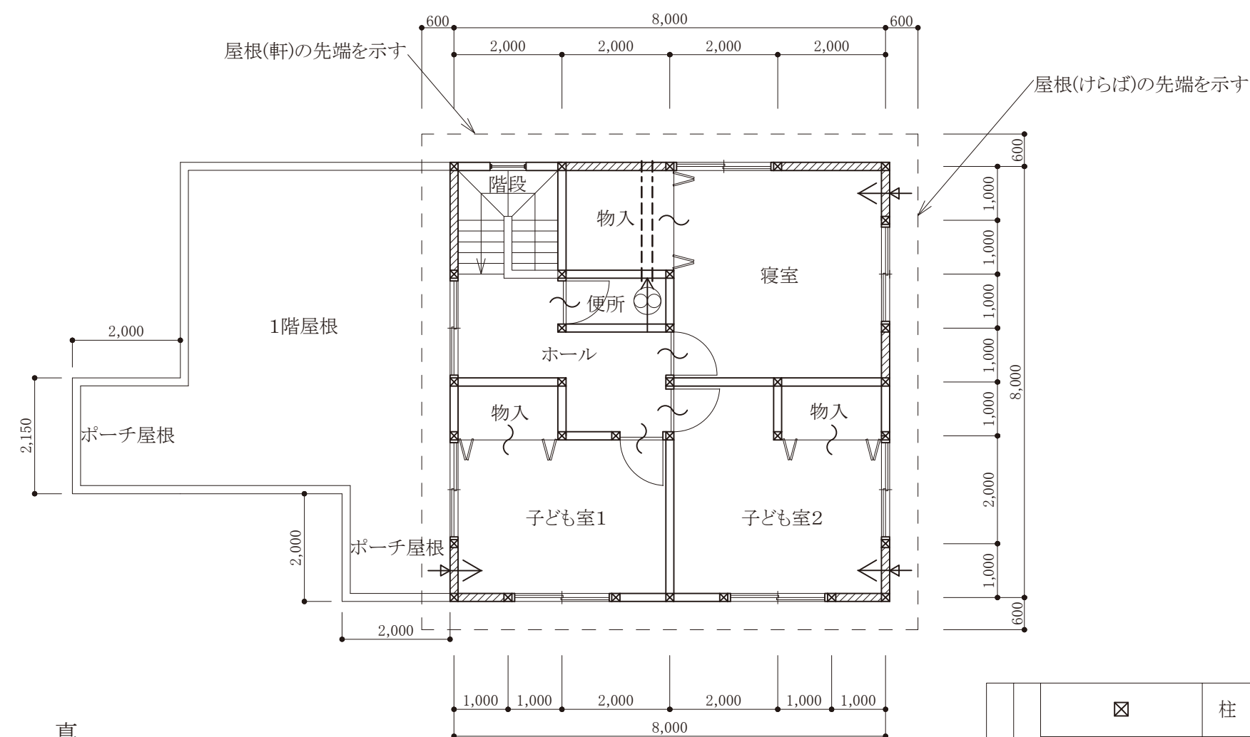
2階平面図
