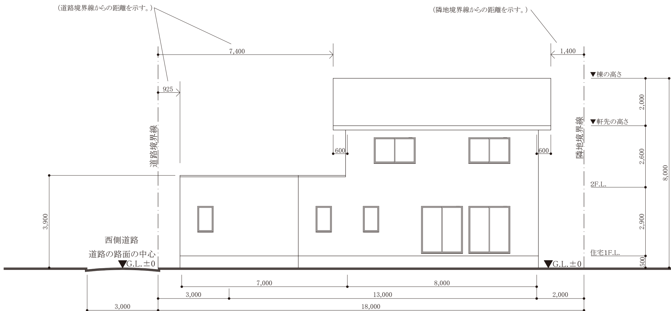
南側立面図
