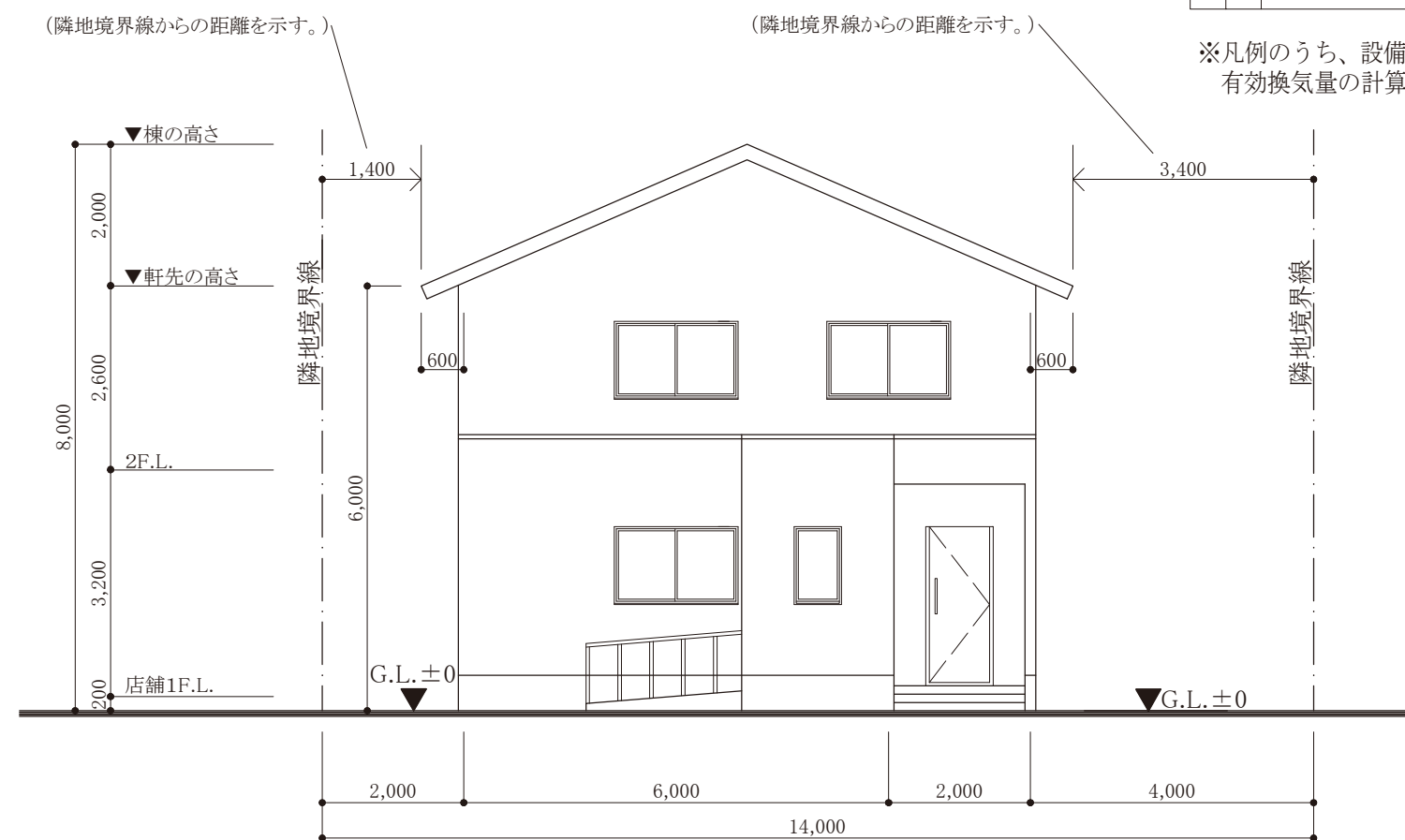
西側立面図
