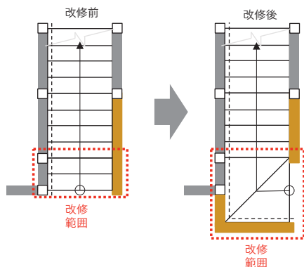
図1 階段改修イメージ
