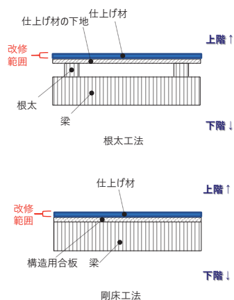
図1 横から見た断面図
