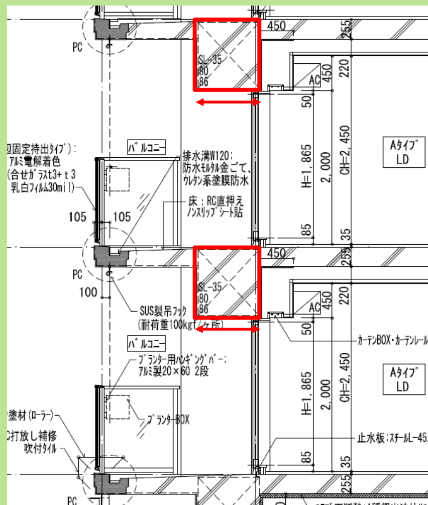
耐震等級 1 の板状マンションの断面図
