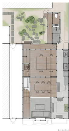
1階平面図
