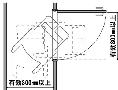
出入口付近の通路の有効幅員が 800mm 以上の場合
