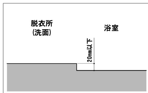
浴室出入口の段差（断面）
