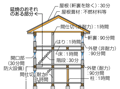
延焼防止建築物（外90分間・内1時間・30分間防火設備） （令元国交告 194号）
