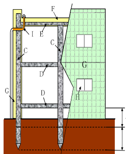
2階建ての場合の骨組（壁、床版）等の構成
