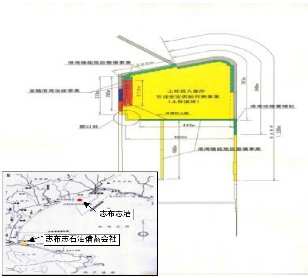
概要図
