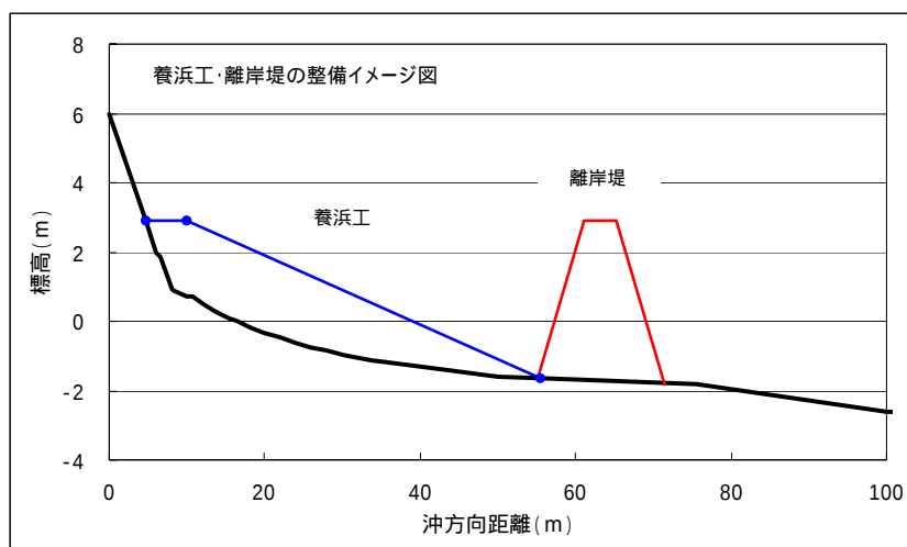
E地区における養浜工・離岸堤の整備イメージ
