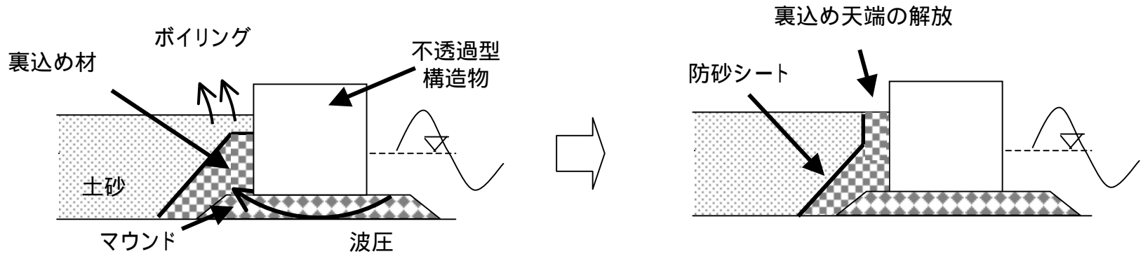
図4 裏込め材設置に伴うボイリングの防止対策
