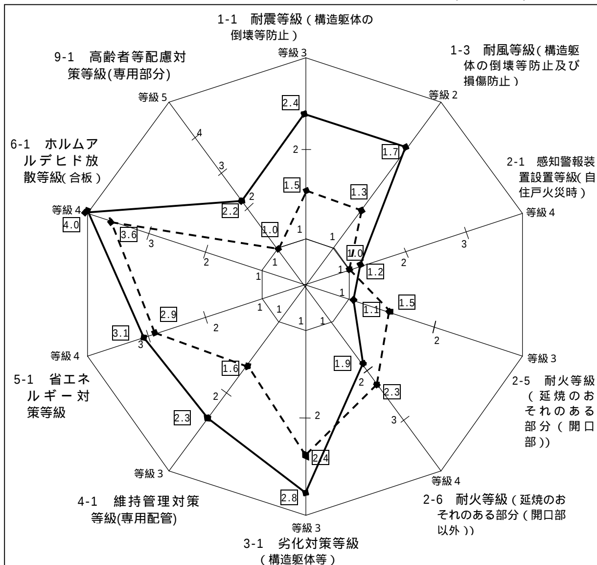
〔住宅性能等級チャート図〕
