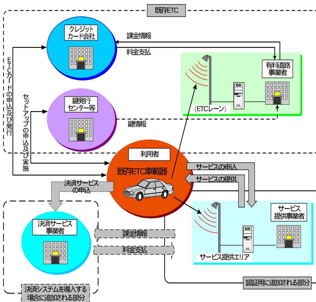
図2 「既存 ETC 車載器の一部機能を活用する場合」の概念図
