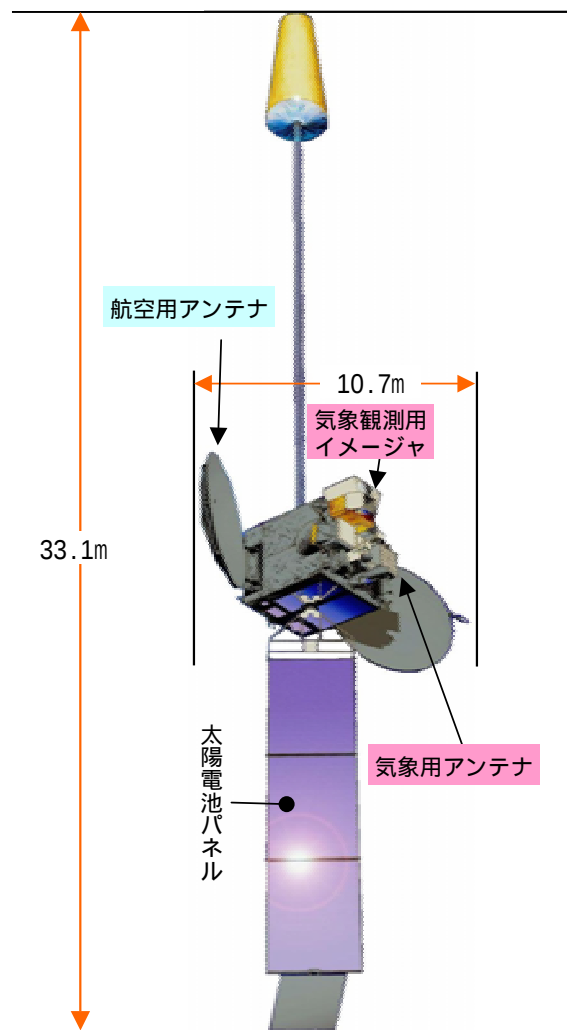
MTSAT展開図
