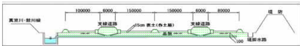
調整関連事業 標準横断面図
