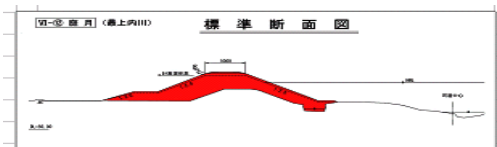
調整関連事業 標準横断面図
