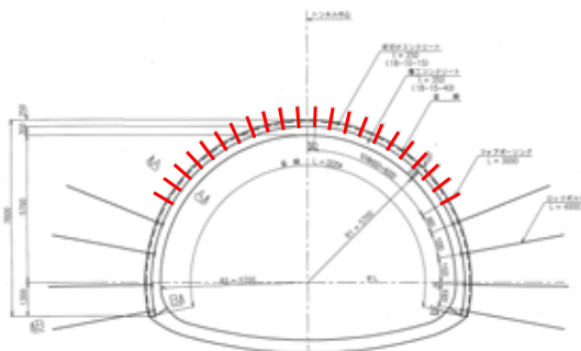
トンネル工 標準断面図
